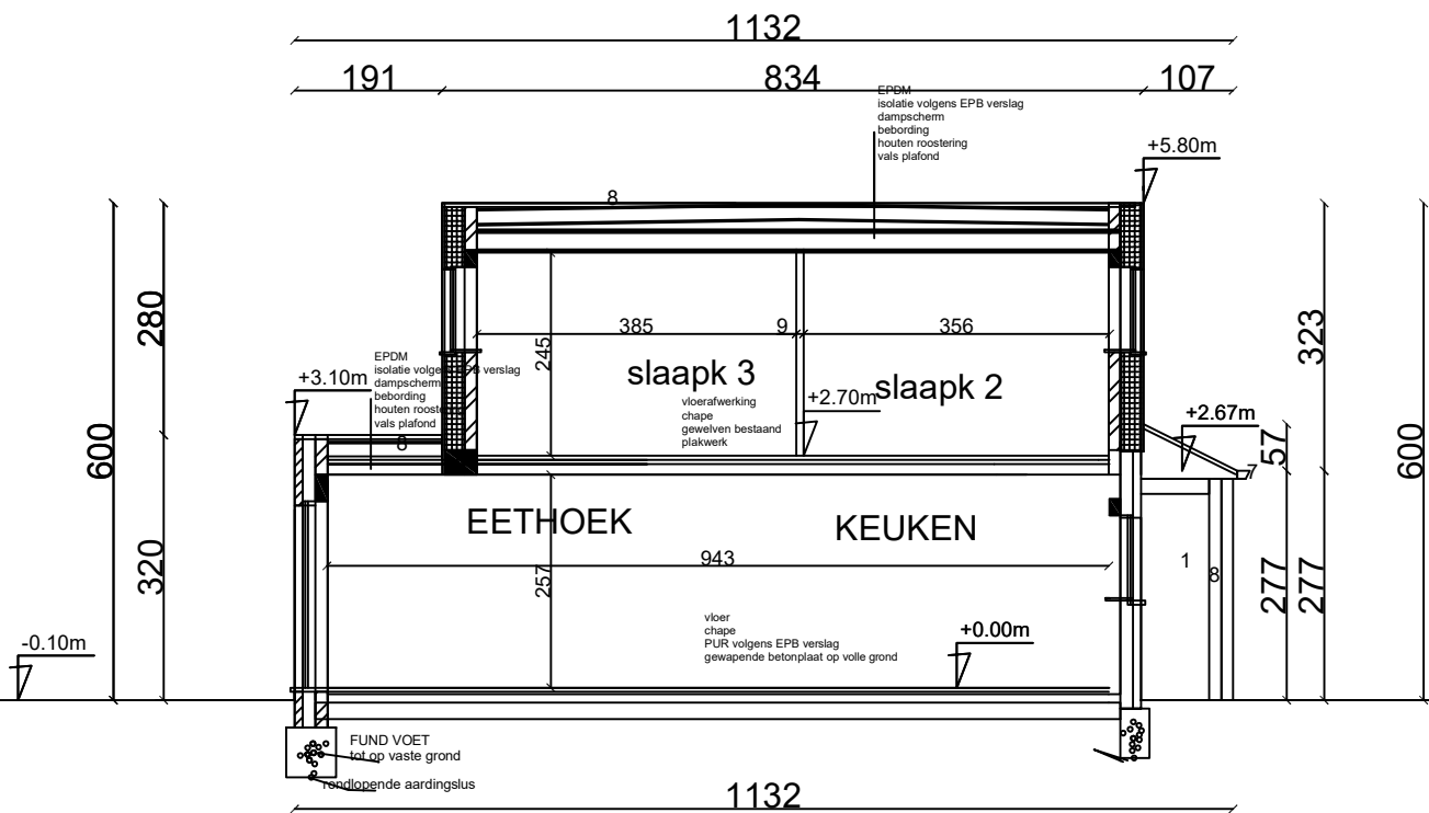
DOORSNEDE AB 1/100
