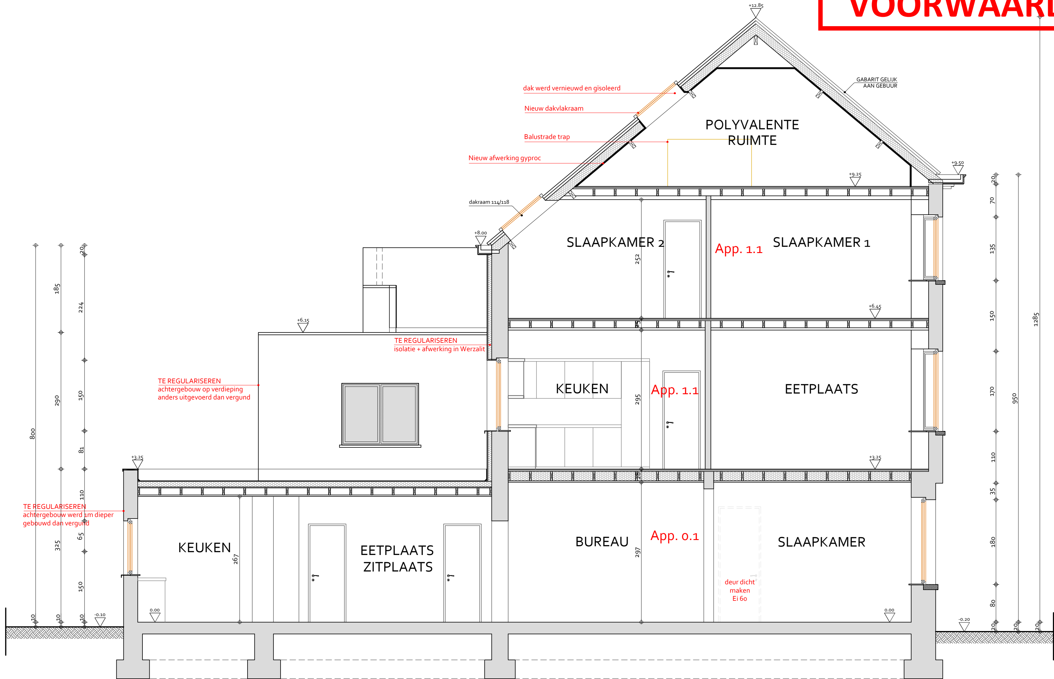
Schaal 1: 50 nieuwe toestand DOORSNEDE BB'
