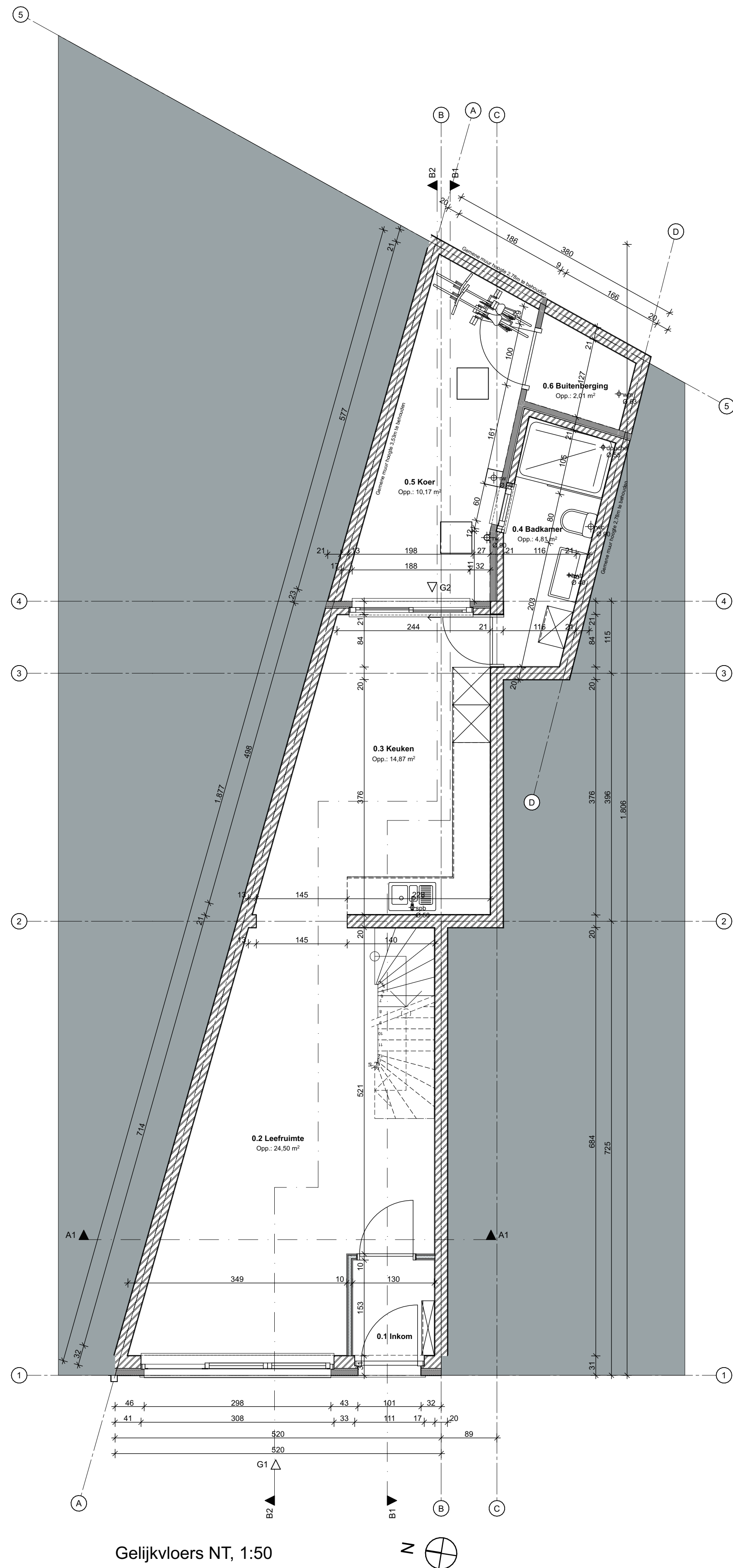
Gelijkvloers NT, 1:50
