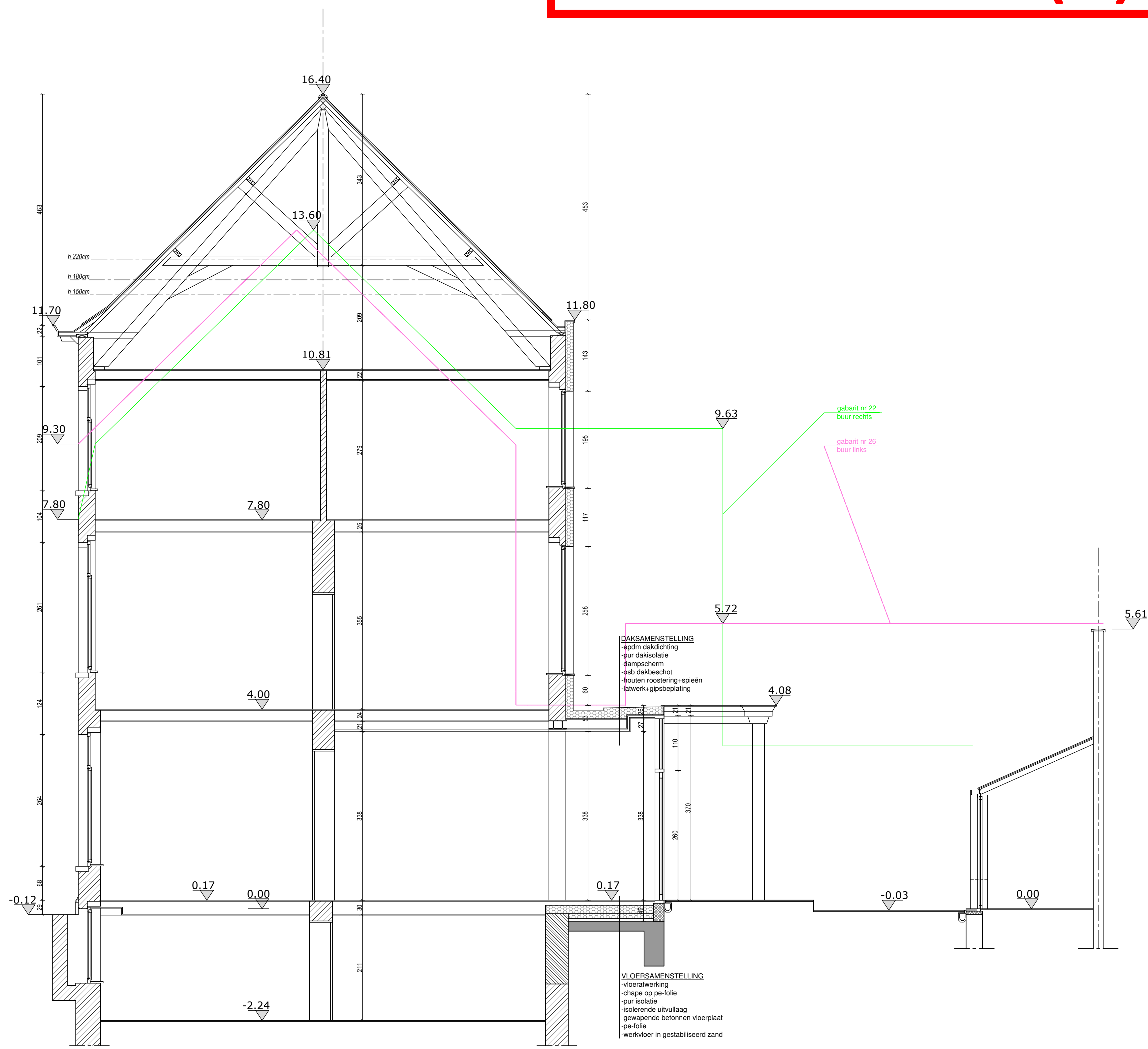
DOORSNEDE B NIEUWE TOESTAND 0 100 200 Schaal 1/50
