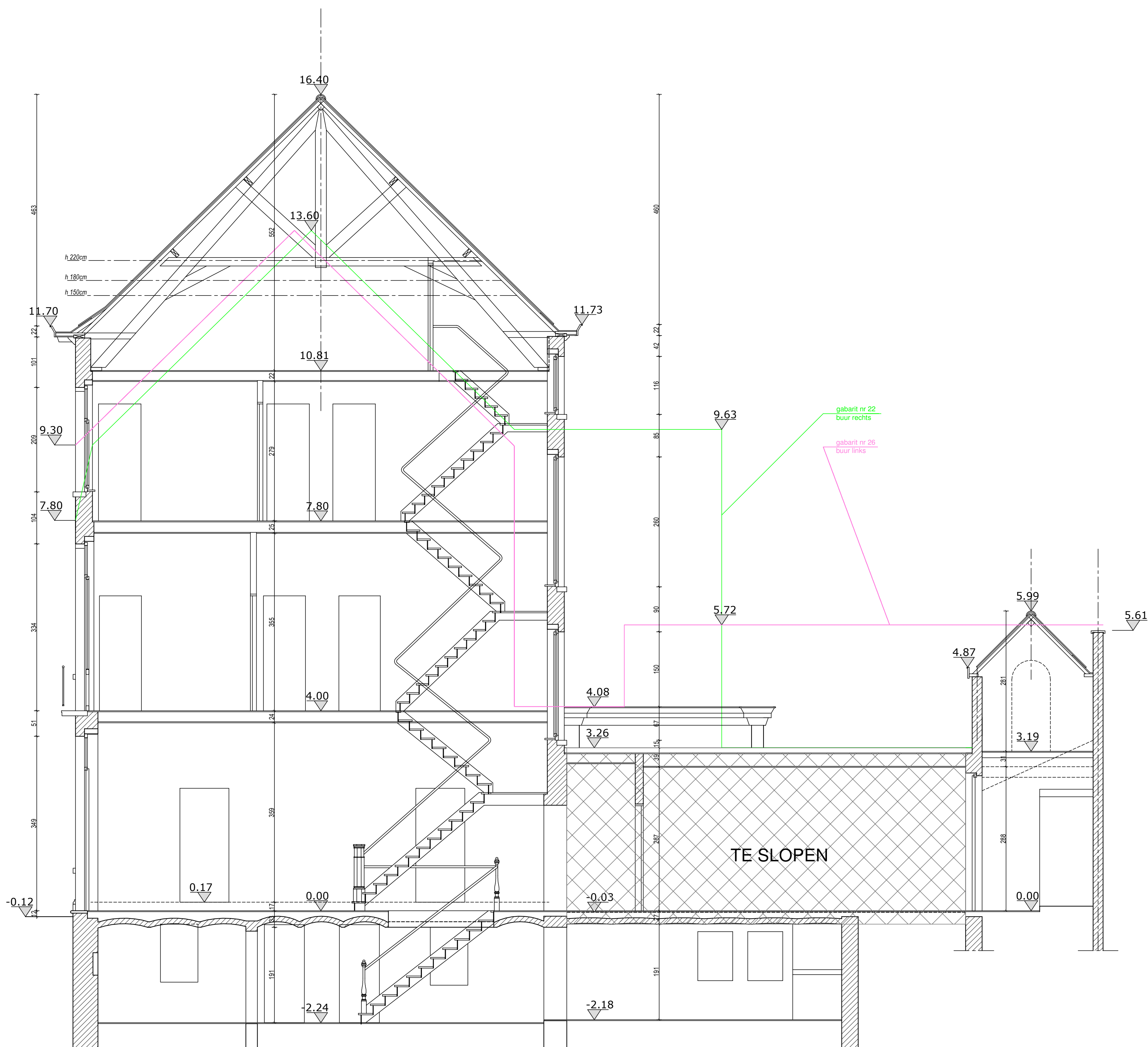
DOORSNEDE A BESTAANDE TOESTAND
