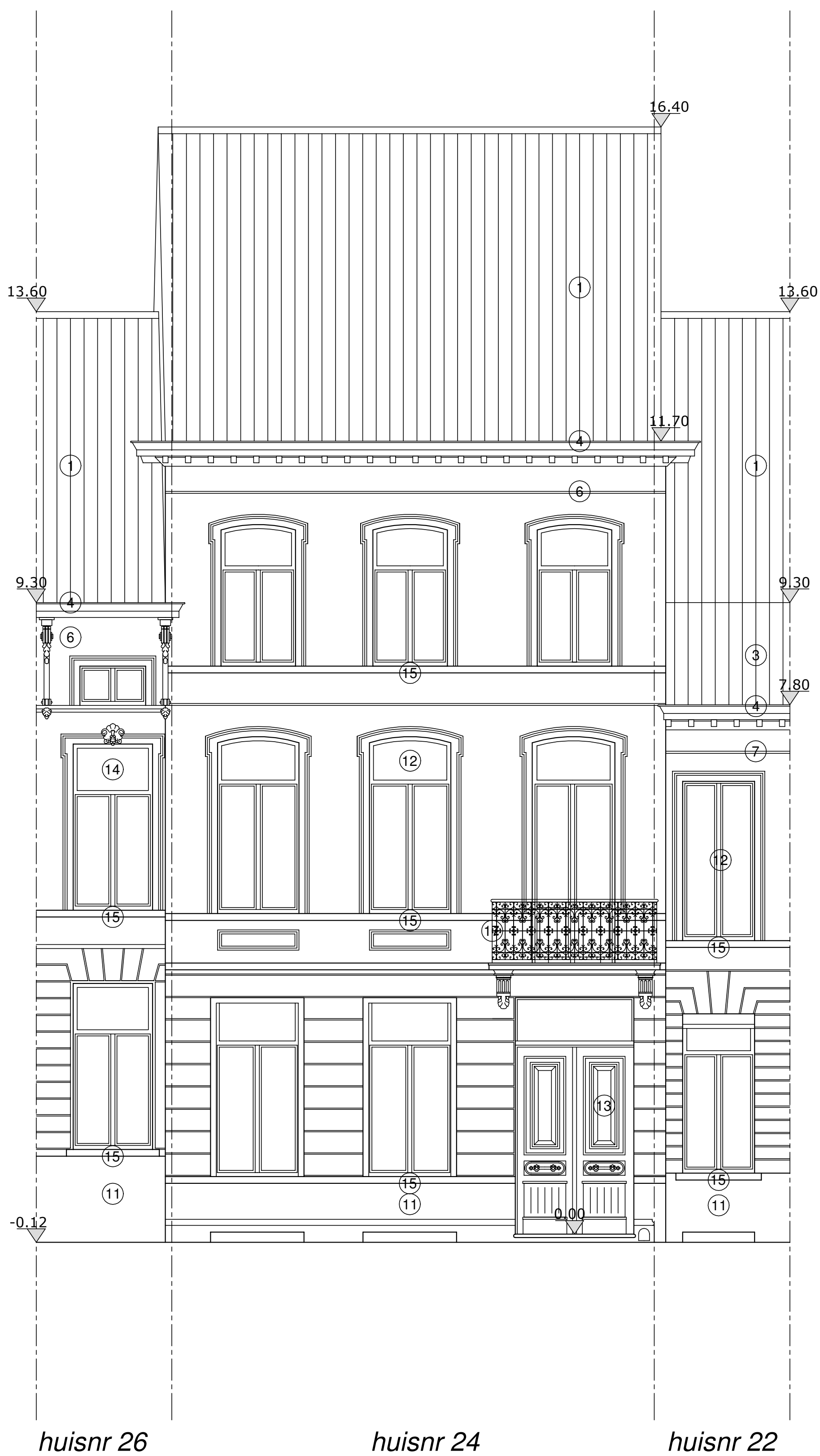
VOORGEVEL BESTAANDE TOESTAND 0 100 200 Schaal 1/50
