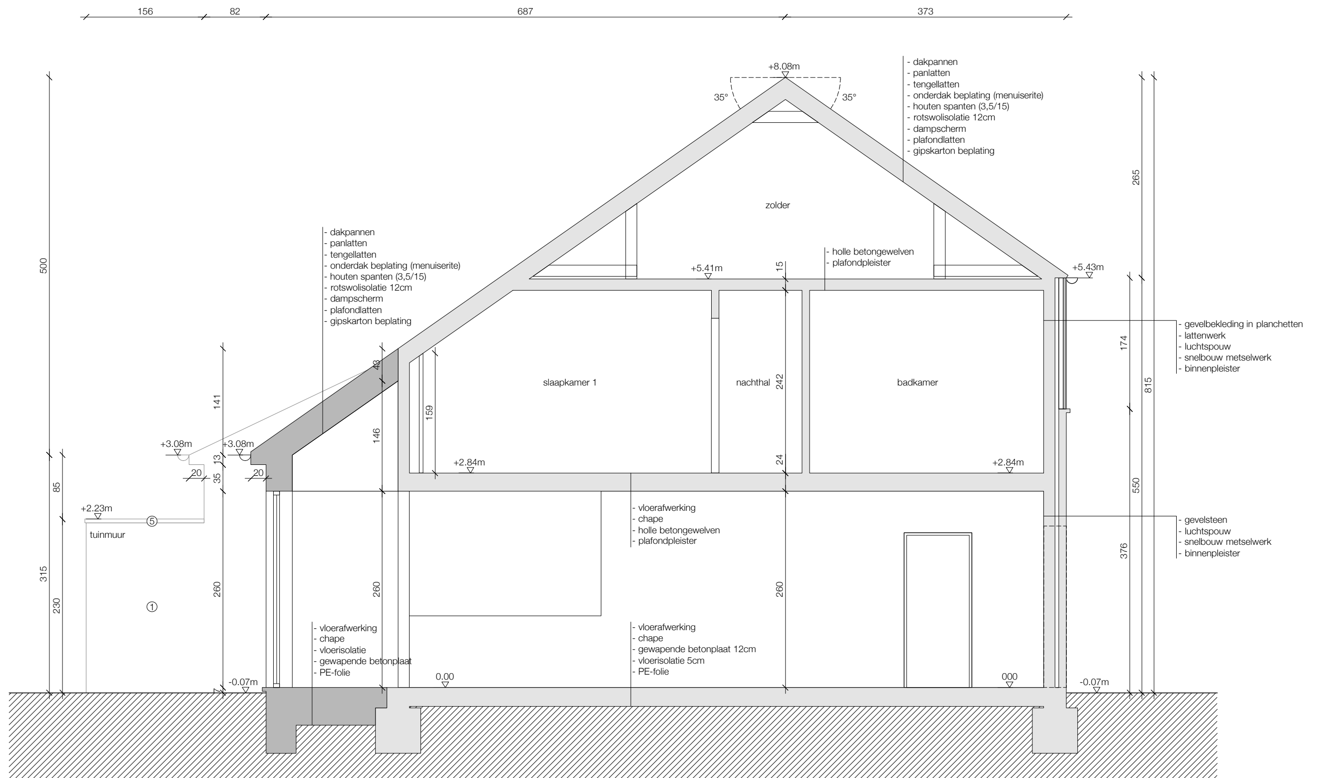
doorsnede AA - schaal 1/50 nieuwe toestand
