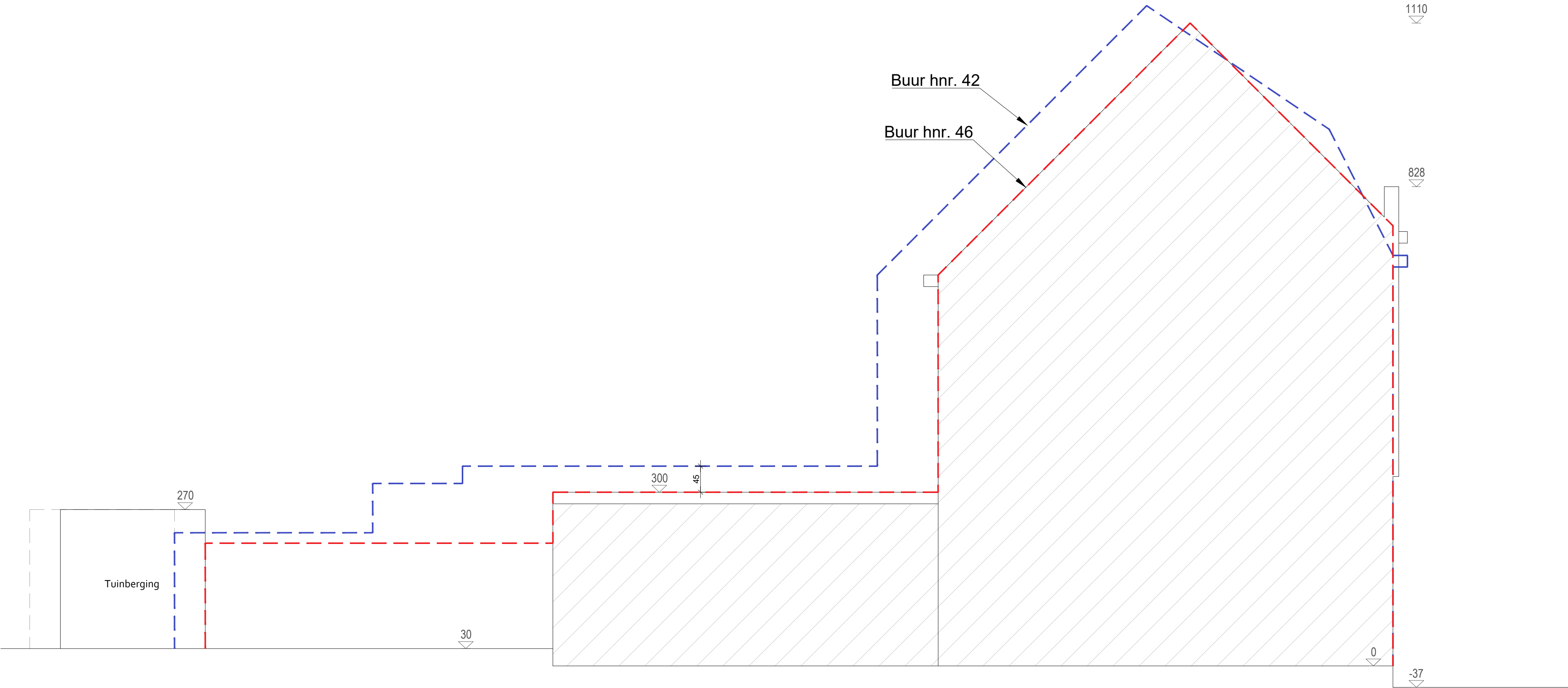
Rechter gevel Bestaande toestand Schaal 1/50
