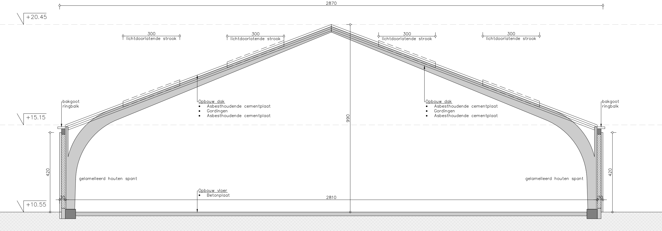
Doorsnede X
