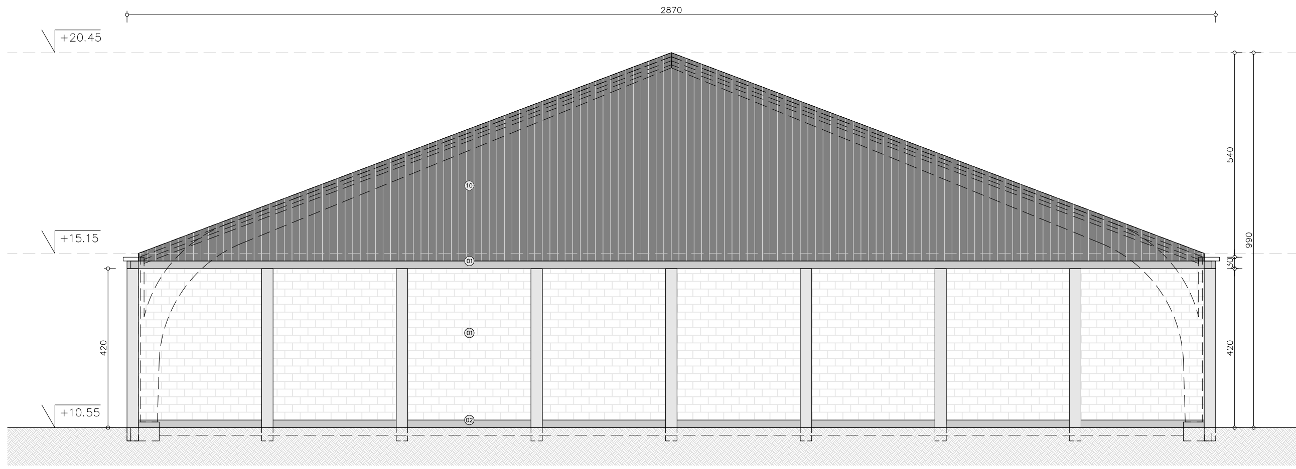
Gevelaanzicht G3
