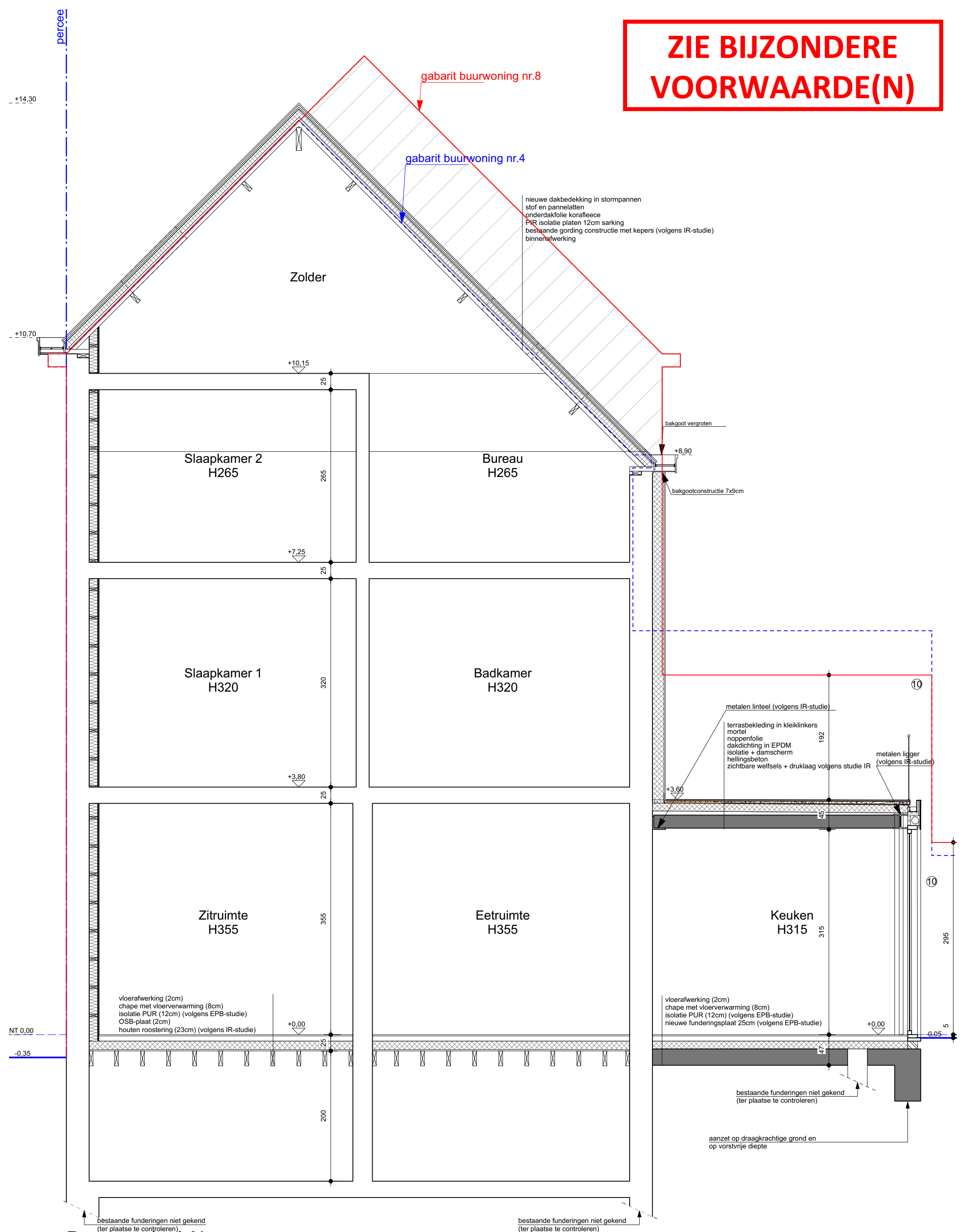
Doorsnede AA' schaal 1/50
