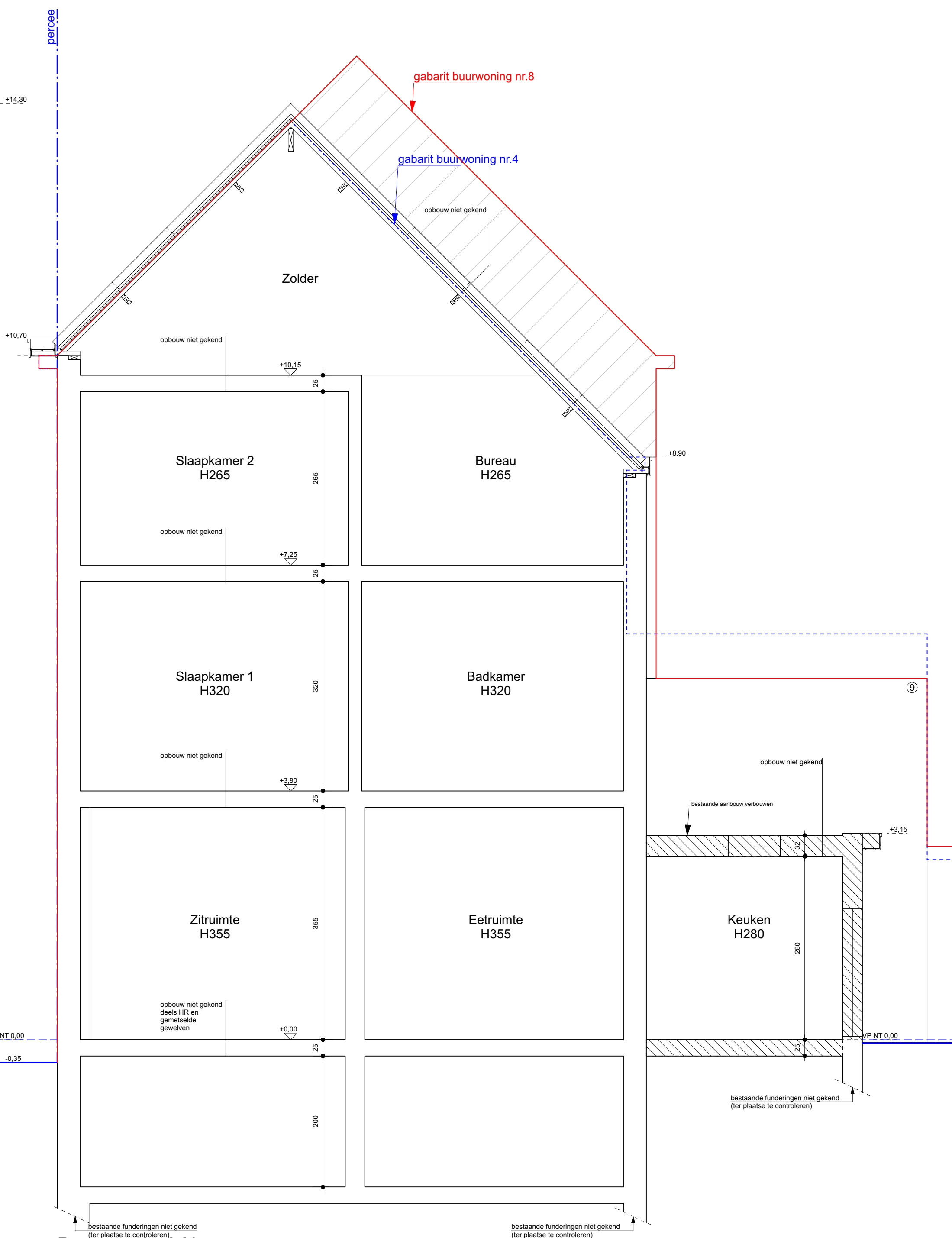
Doorsnede AA' schaal 1/50
