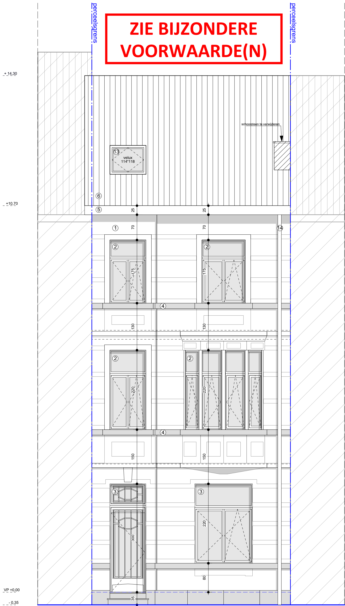
Voorgevel schaal 1/50
