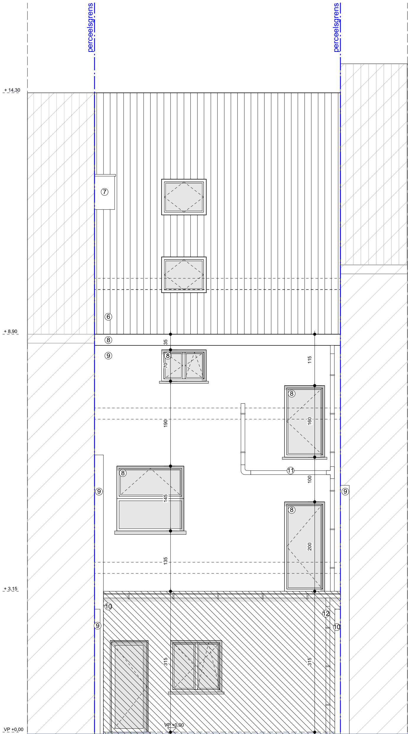
Achtergevel schaal 1/50
