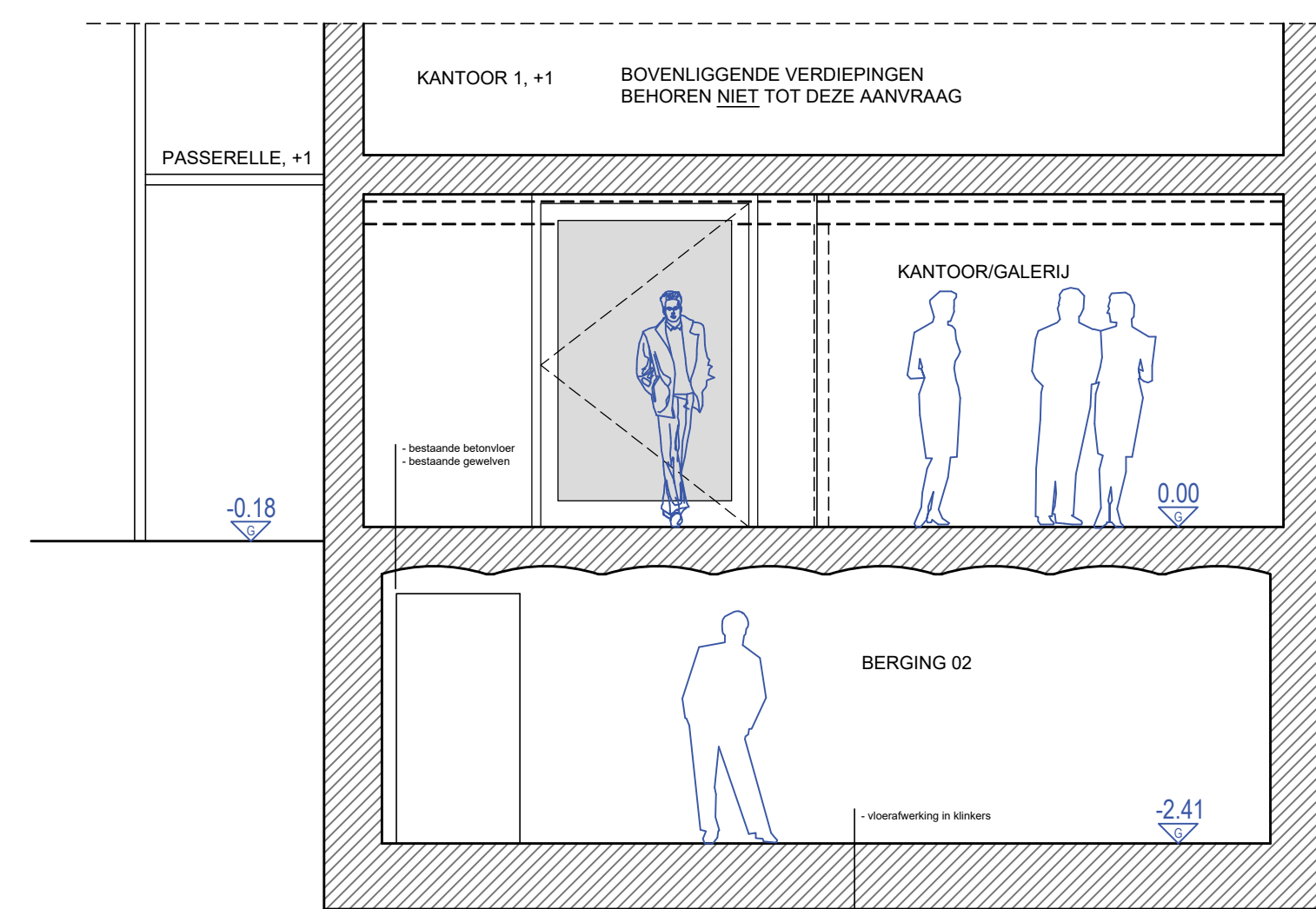
DOORSNEDE BB BT
