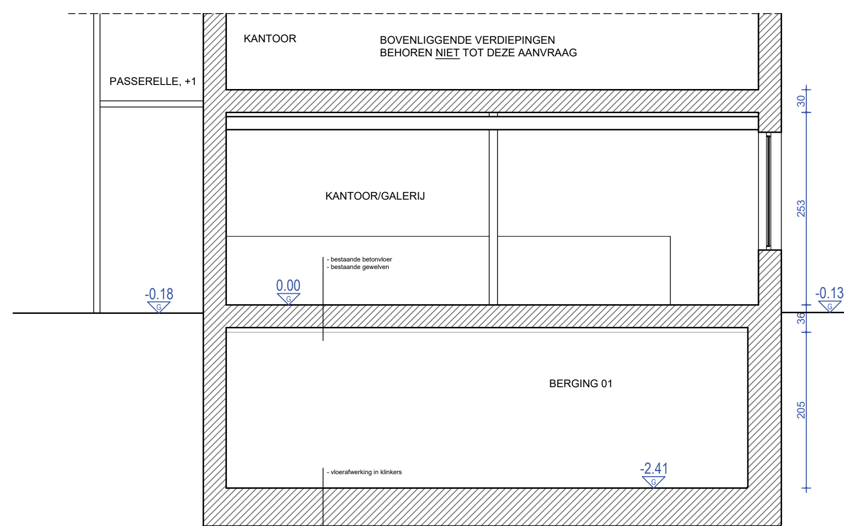
DOORSNEDE CC BT
