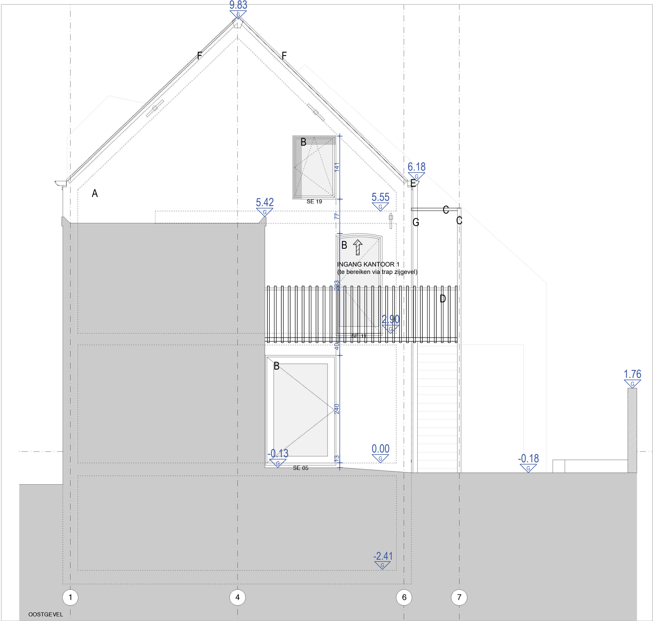
GEVEL OOST NT (ongewijzigd )
