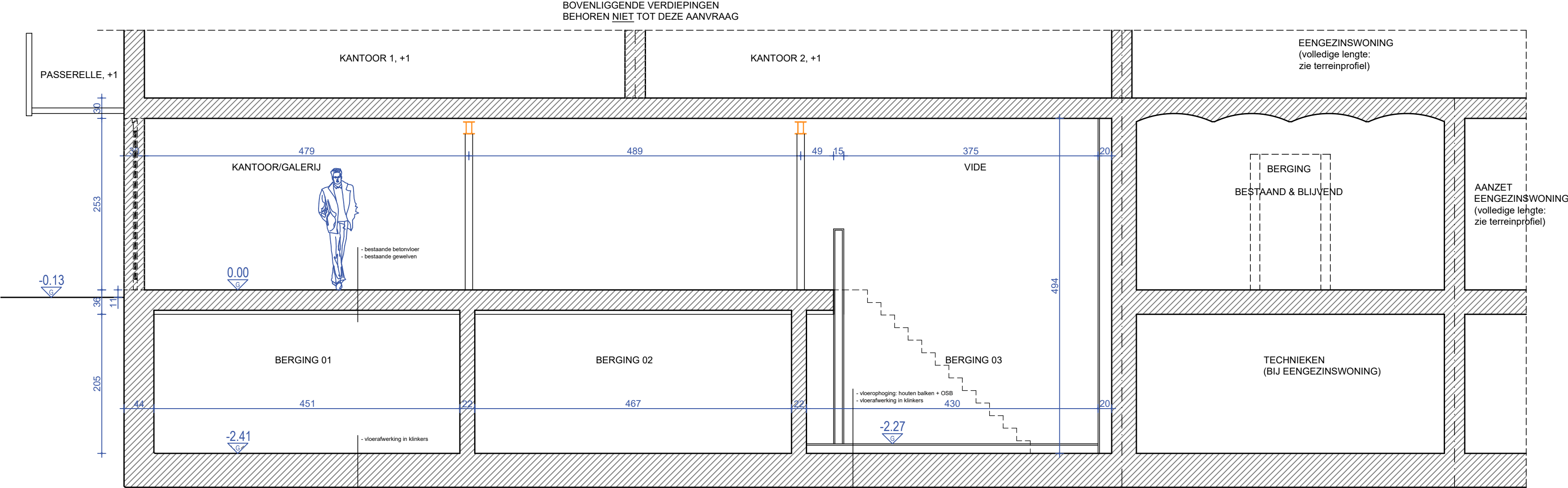
DOORSNEDE AA BT
