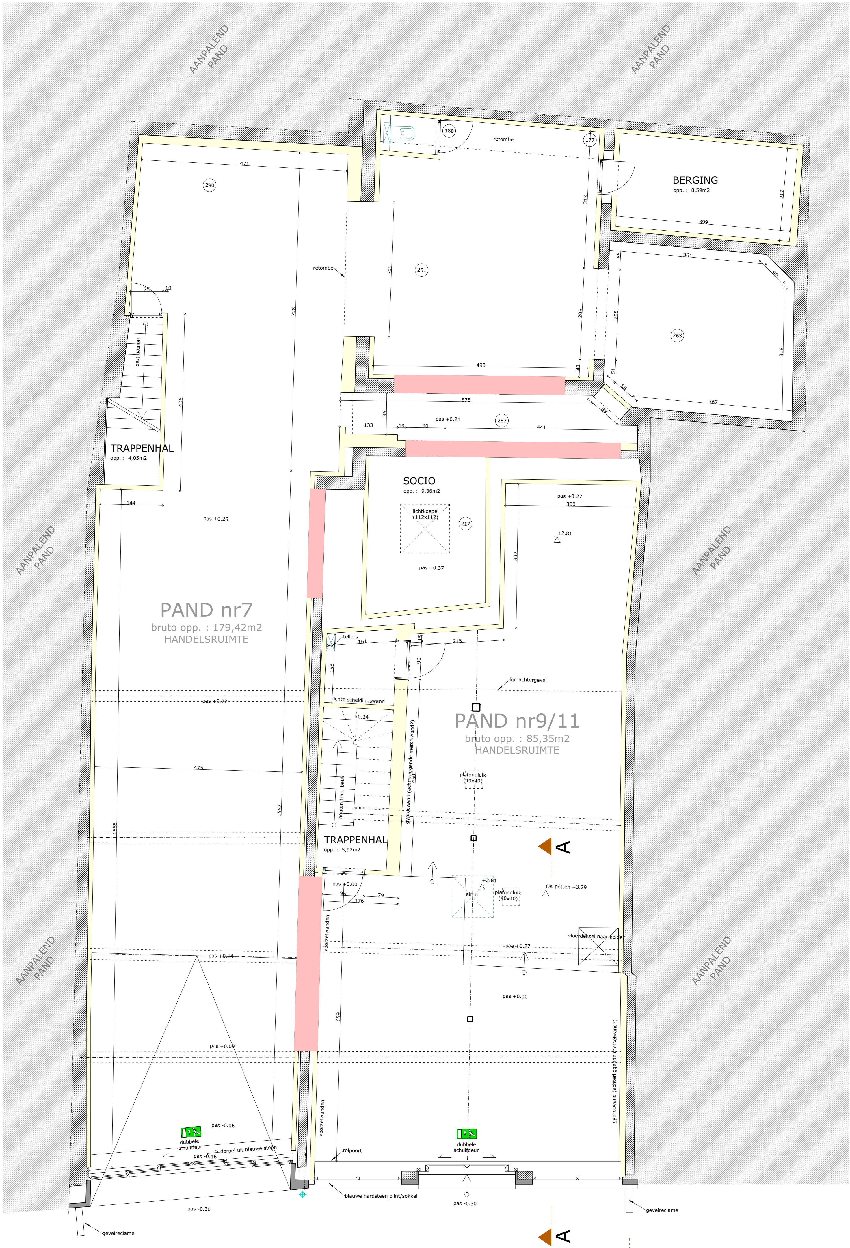
GRONDPLAN +0 schaal: 1/50
