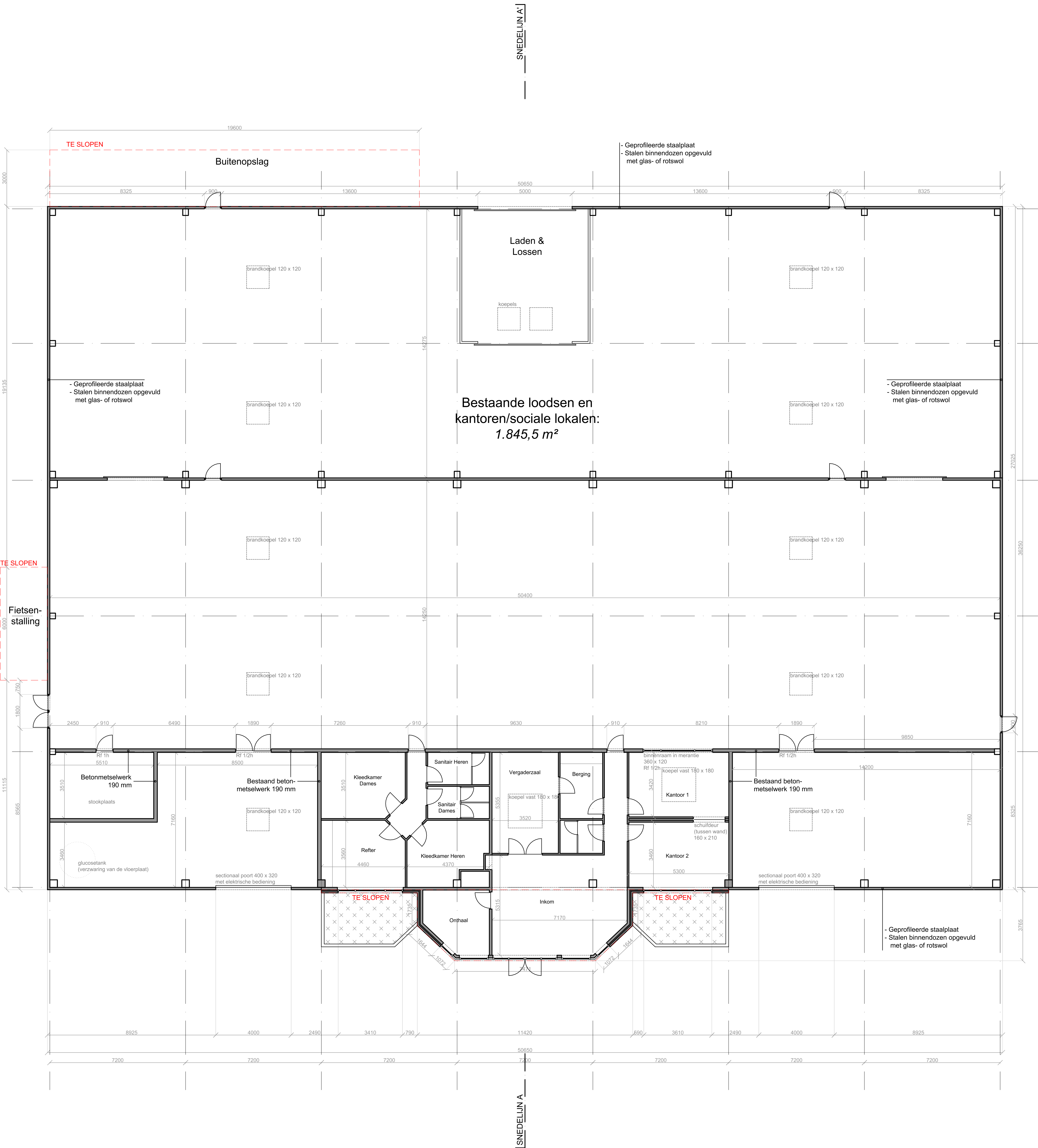
PLAN GELIJKVLOERS Bestaande situatie
