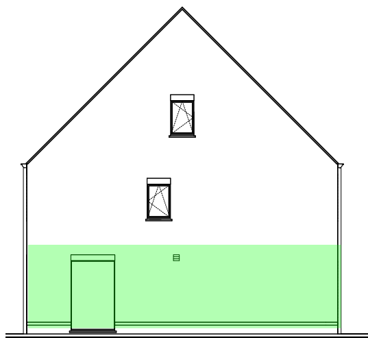
Zijgevel rechts
