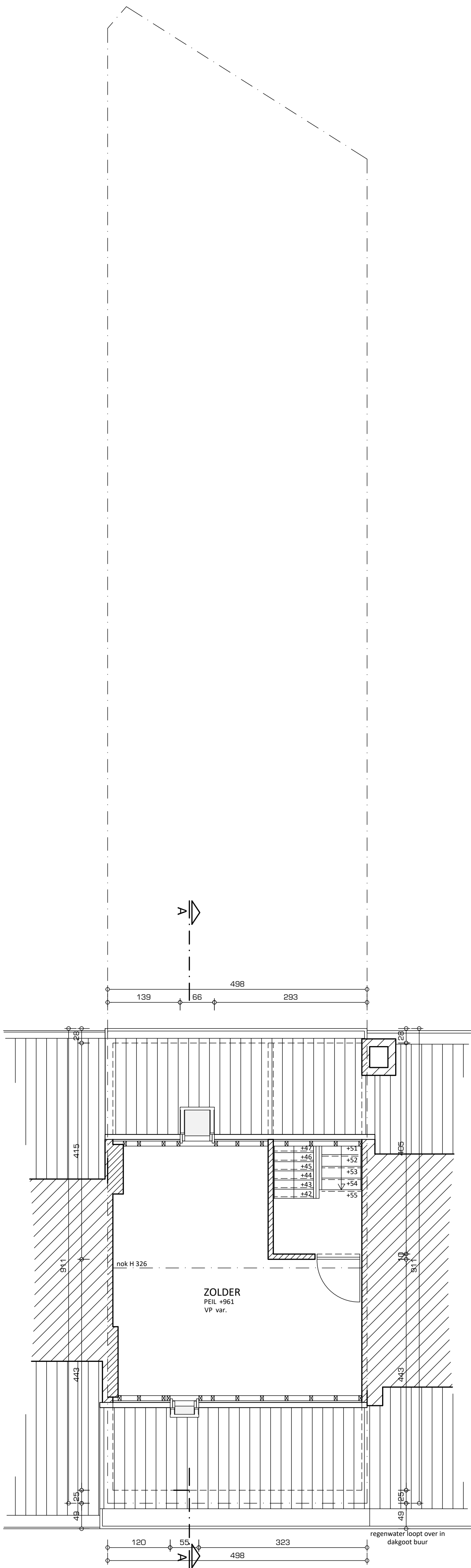
ZOLDER horizontale snede op H160cm (tov Peil +961)
