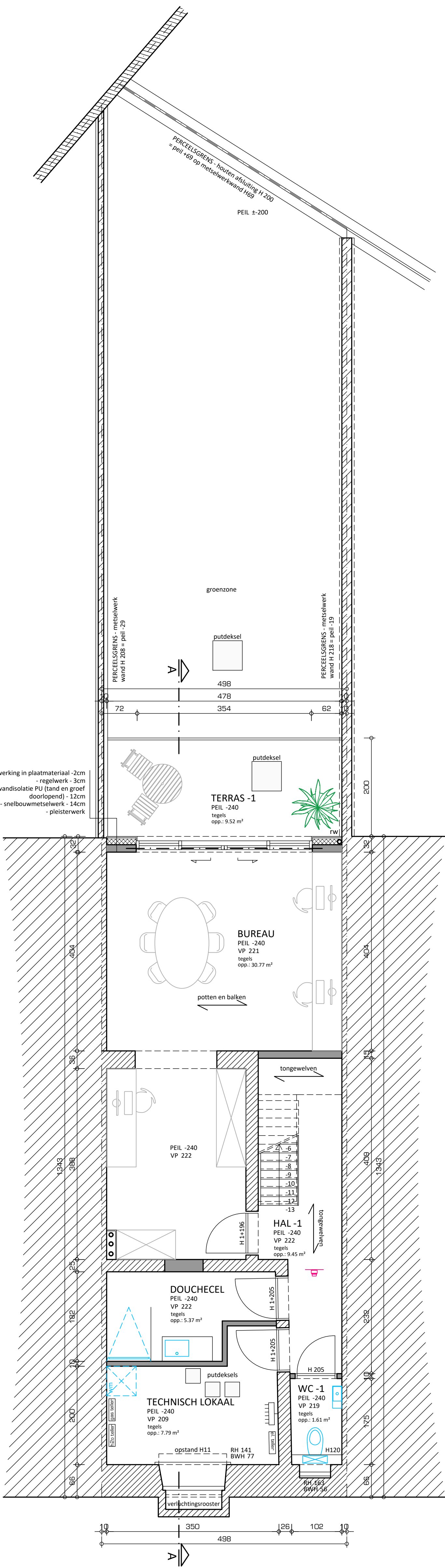
KELDERVERDIEPING
