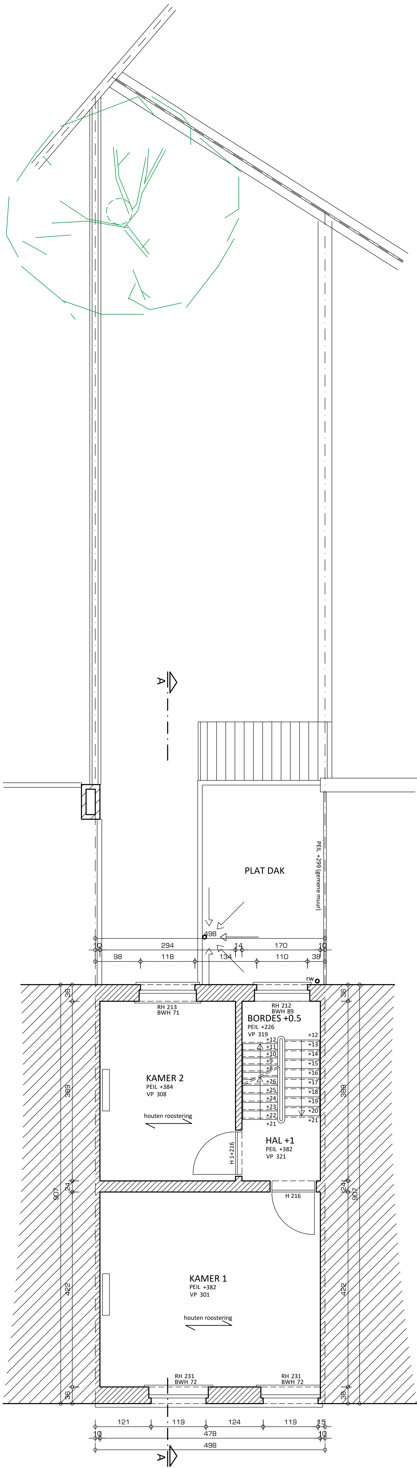
VERDIEPING +1
