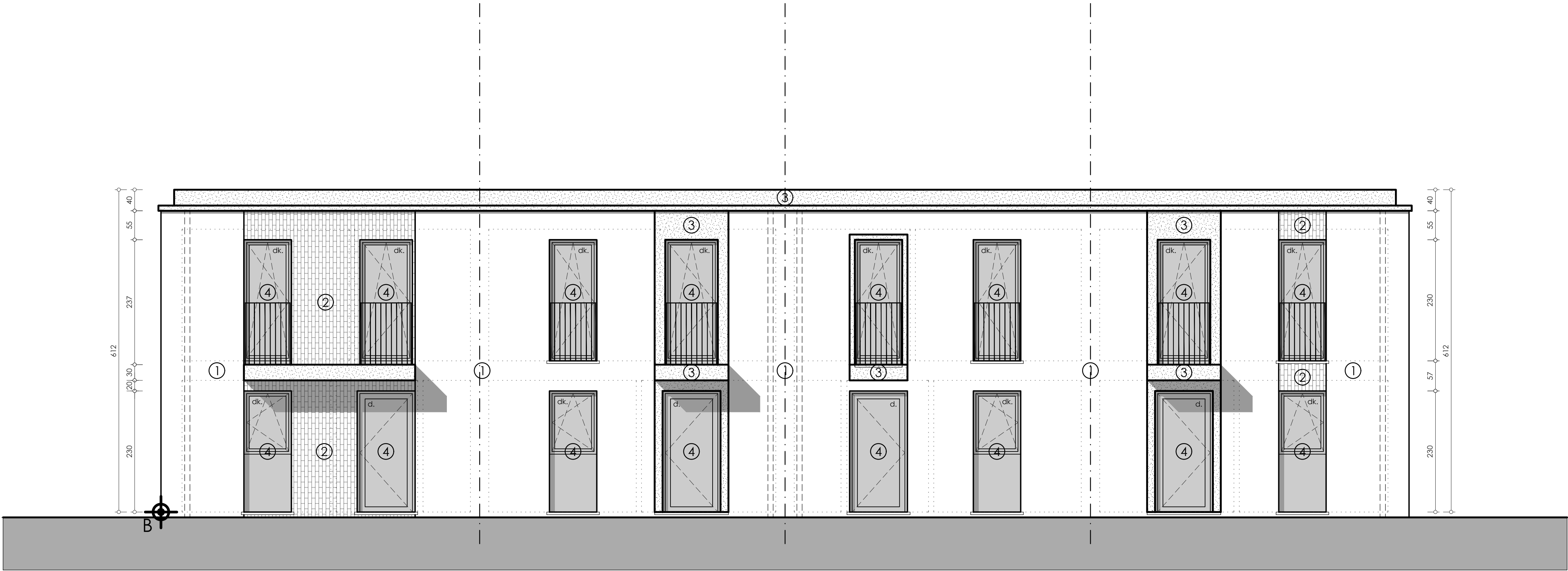
Voorgevel
