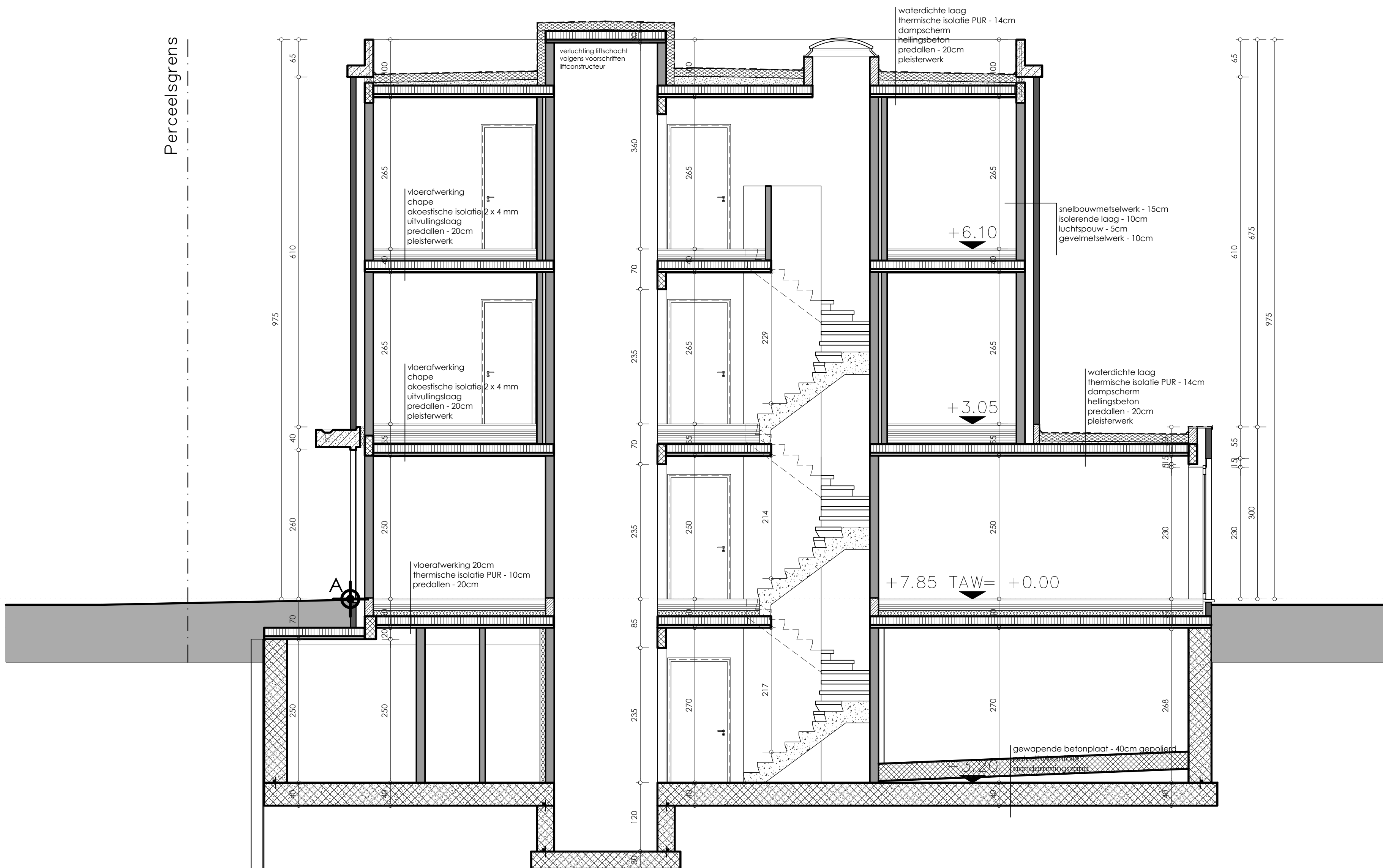
Doorsnede 3-3
