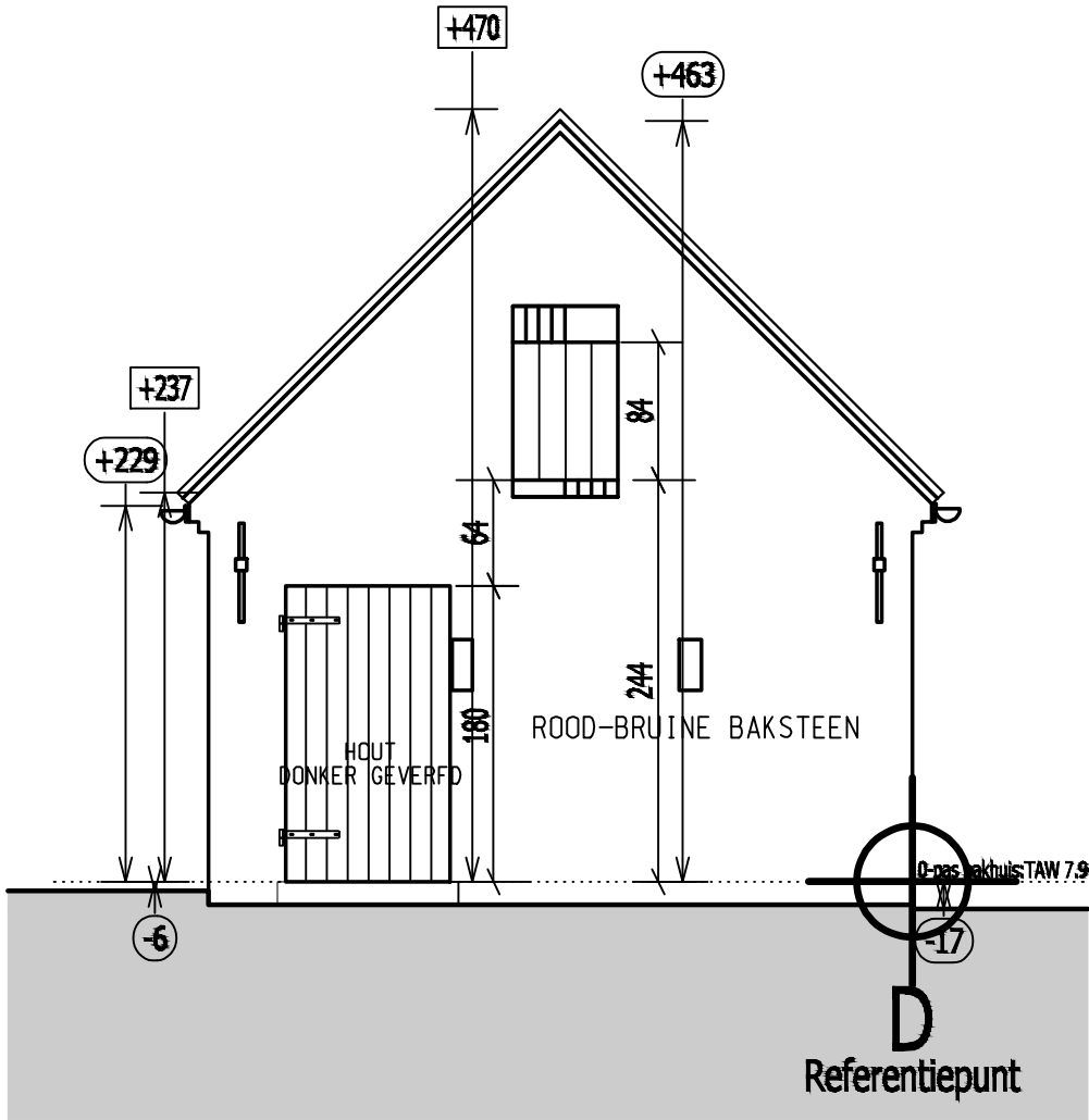
ACHTERGEVEL (D)
