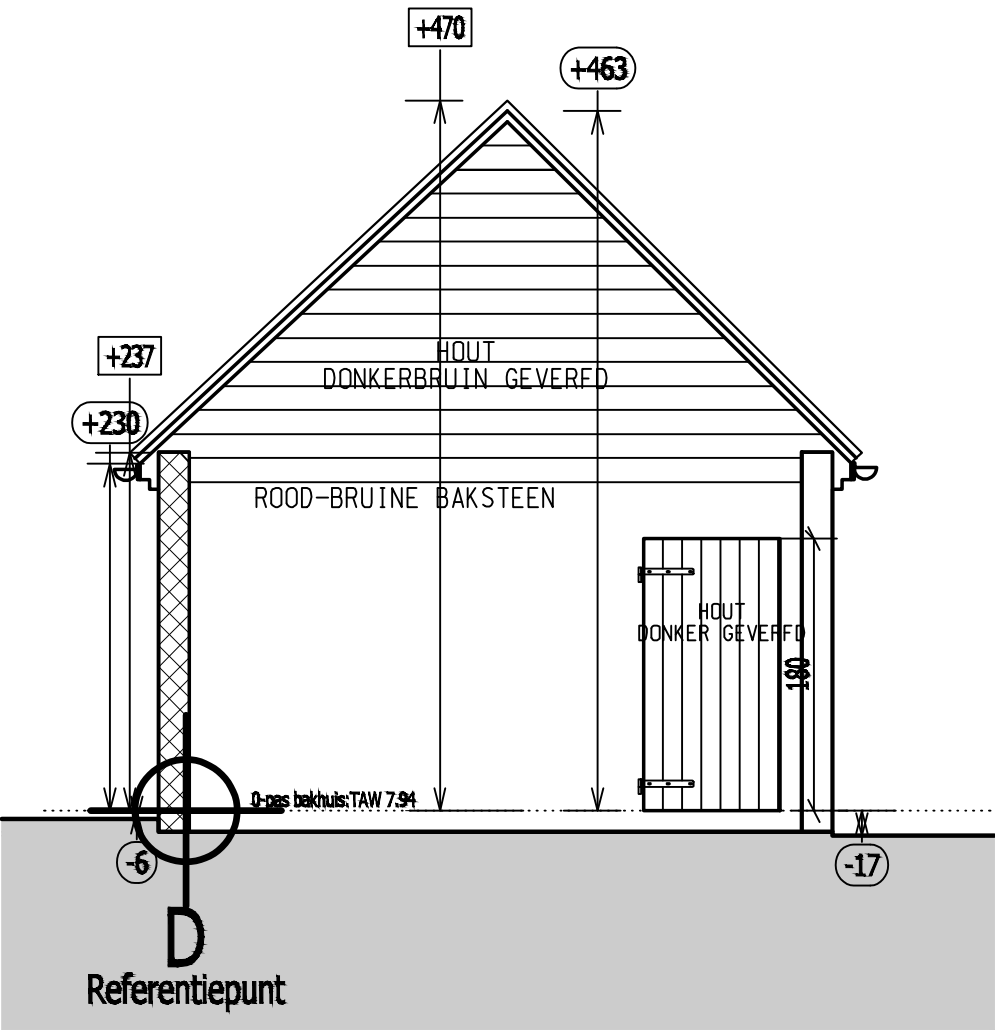
VOORGEVEL (E)
