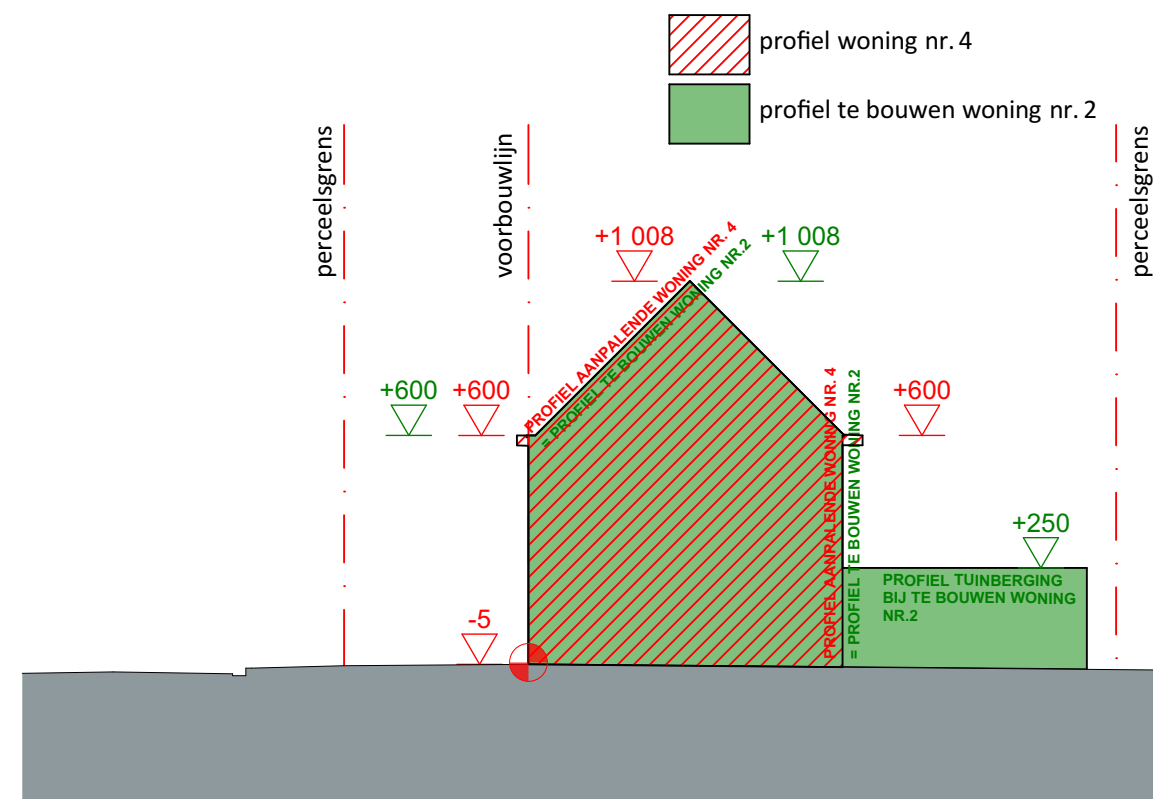
BEBOUWING THV PERCEELSGRENS MET WONING NR. 4 nieuwe toestand
