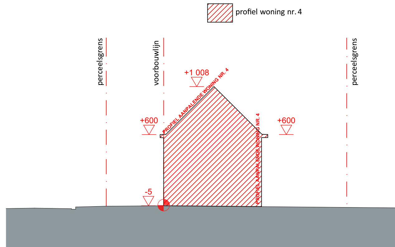
BEBOUWING THV PERCEELSGRENS MET WONING NR. 4 bestaande toestand
