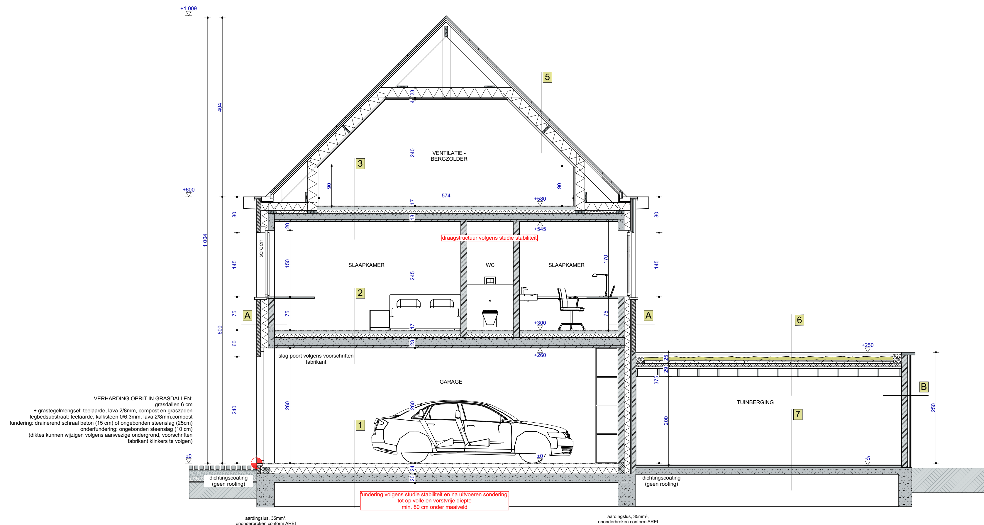
SNEDE AA 1:50
