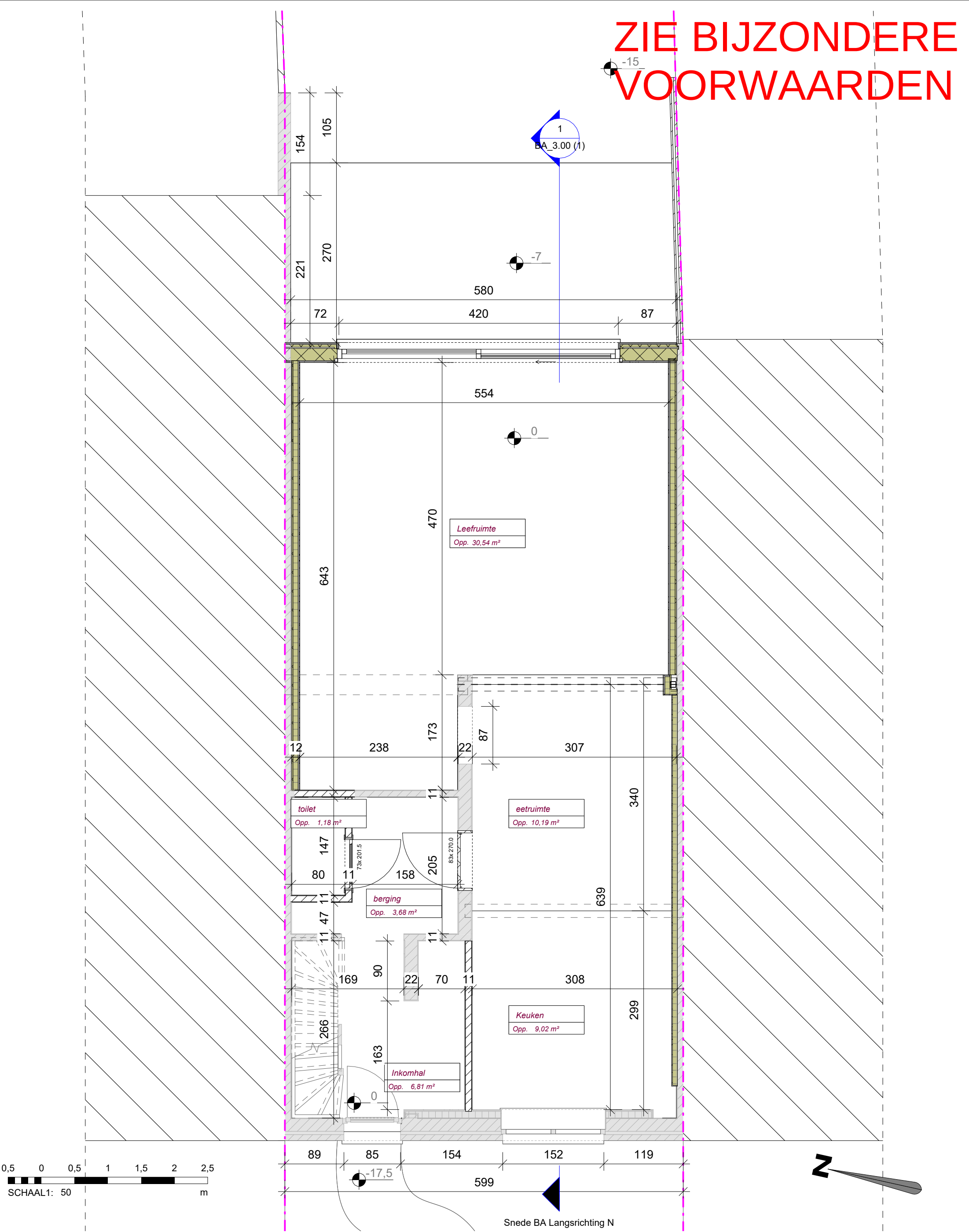
BA_1.00 (1) P_N_1.00_Grondplan Gelijkvloers
