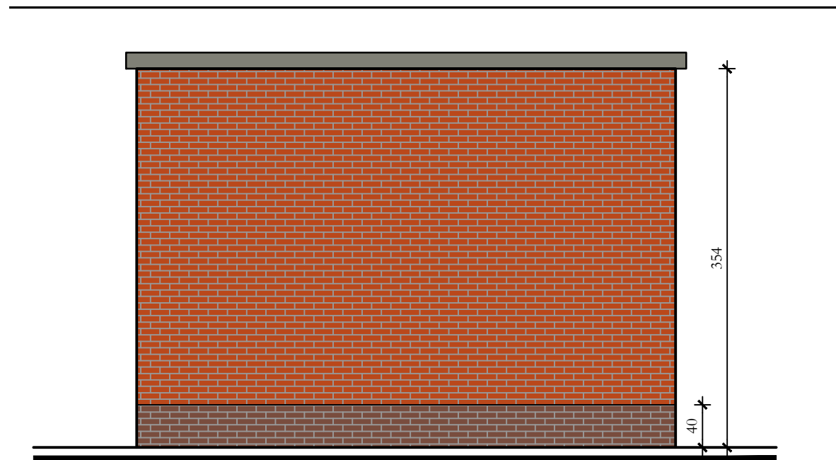
ACHTERGEVEL Bestaande Cabine OP SCHAAL 1 / 50
