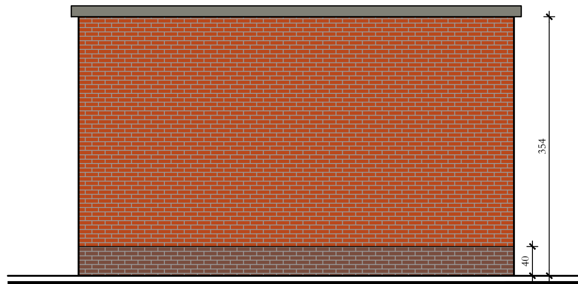
ZIJGEVEL LINKS Bestaande Cabine OP SCHAAL 1 / 50
