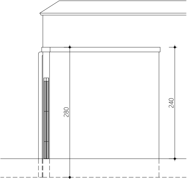
gevel noord tuinhok nieuwe toestand
