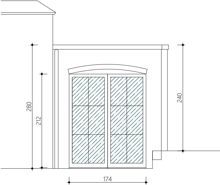
gevel oost tuinhok nieuwe toestand
