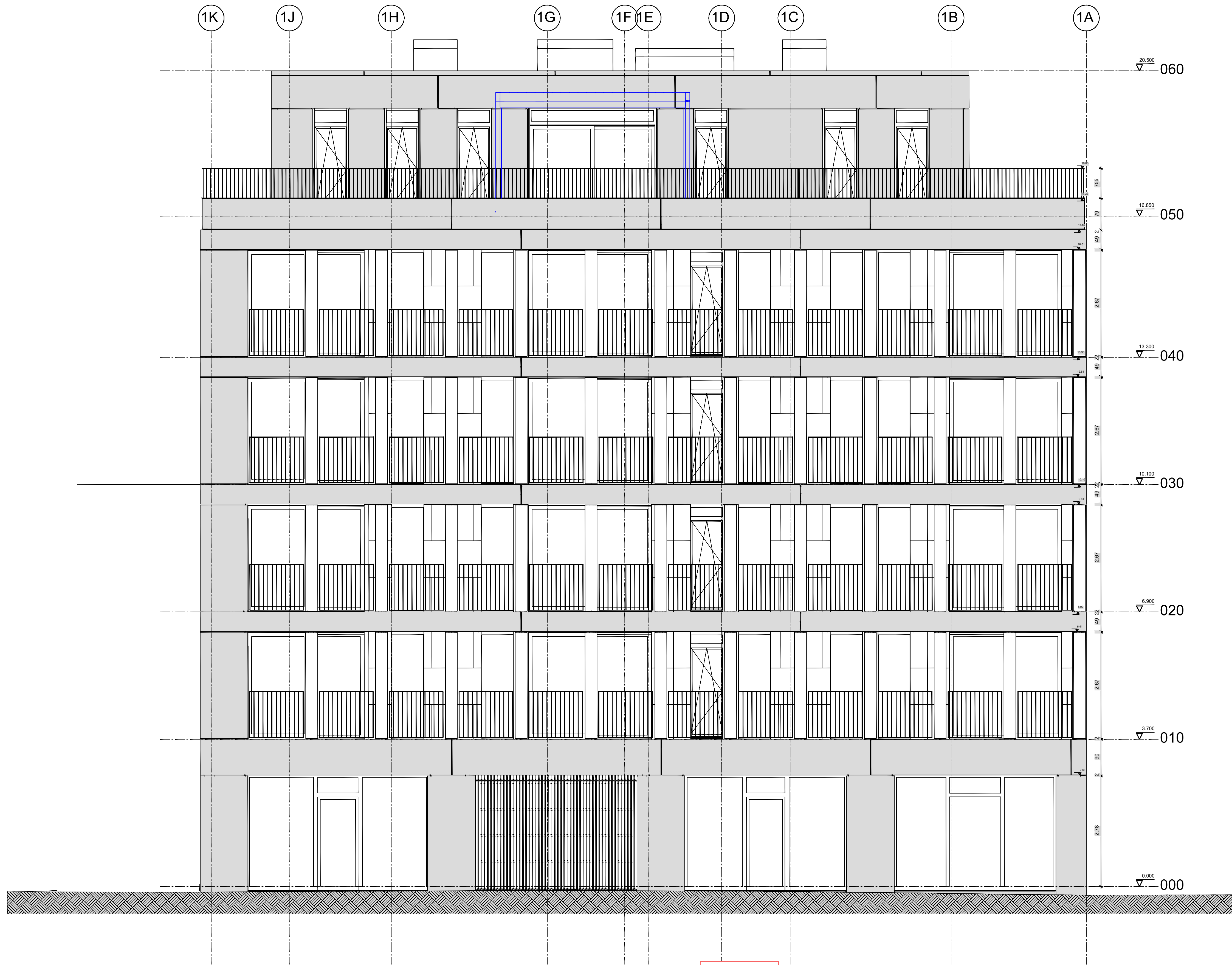
Muishondstraat 2 bus 501 Geveltekening nieuwe toestand
