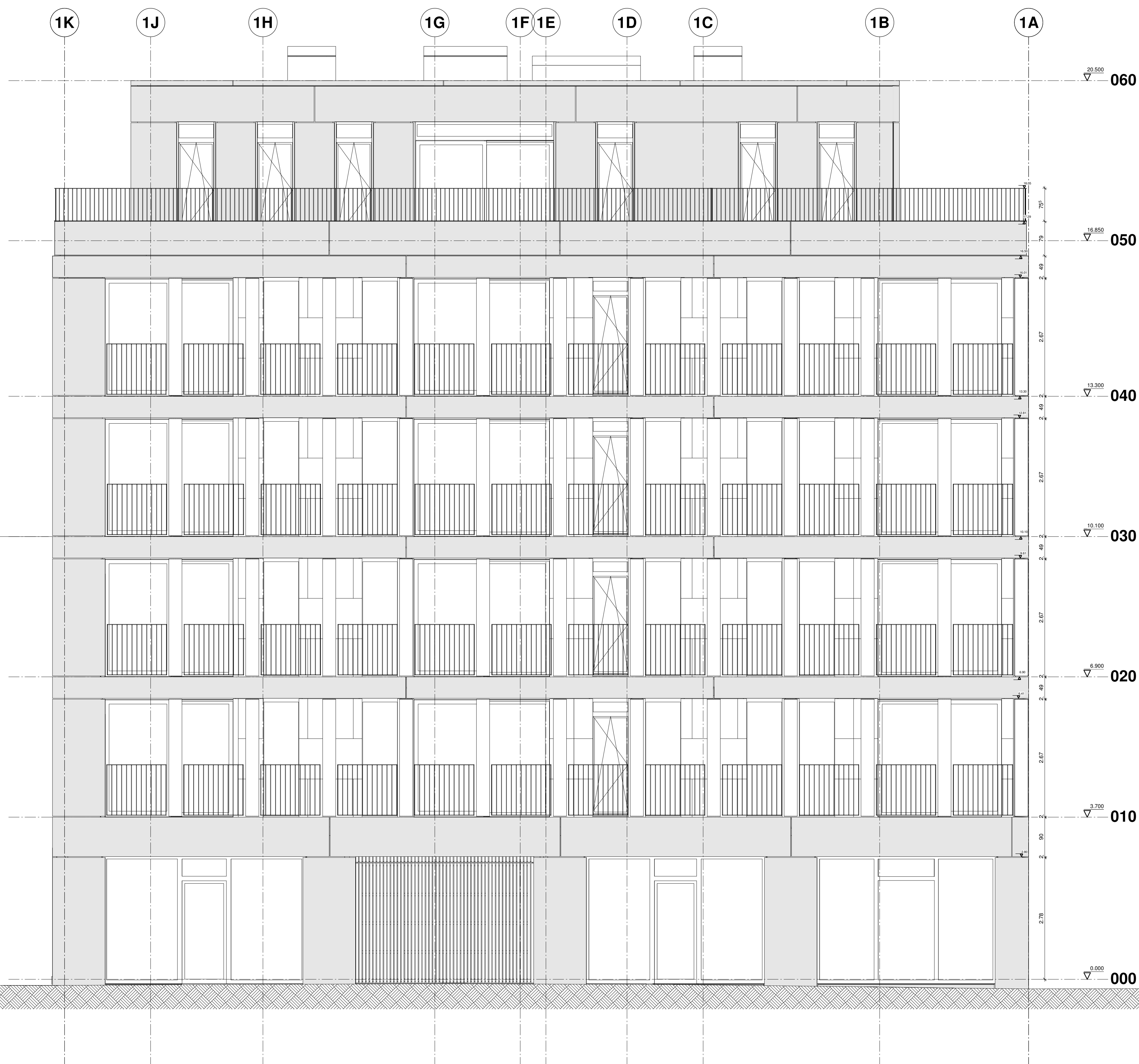
Muishondstraat 2 bus 501 Geveltekening bestaande toestand
