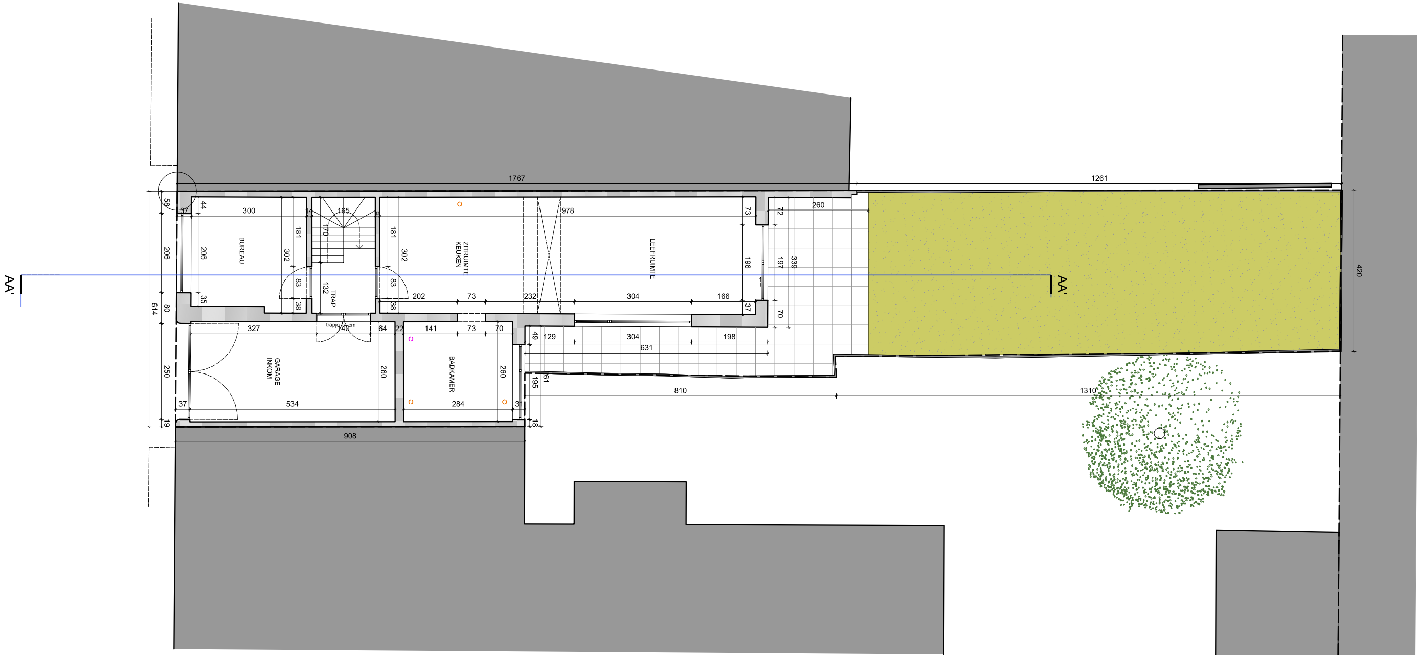
GRONDPLAN VERDIEPING +0 - bestaande toestand
