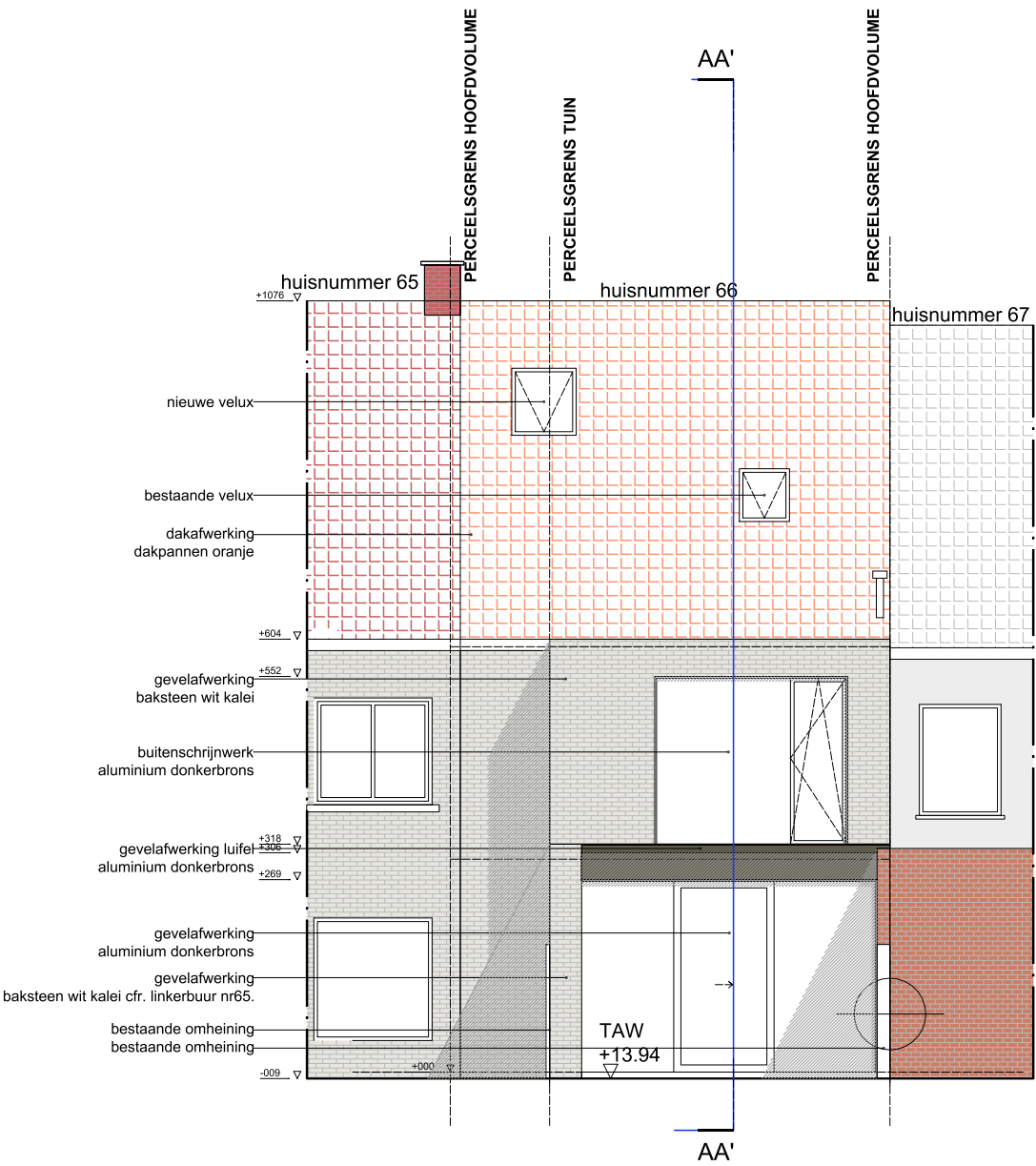
ACHTERGEVEL ZUID-WEST - nieuwe toestand
