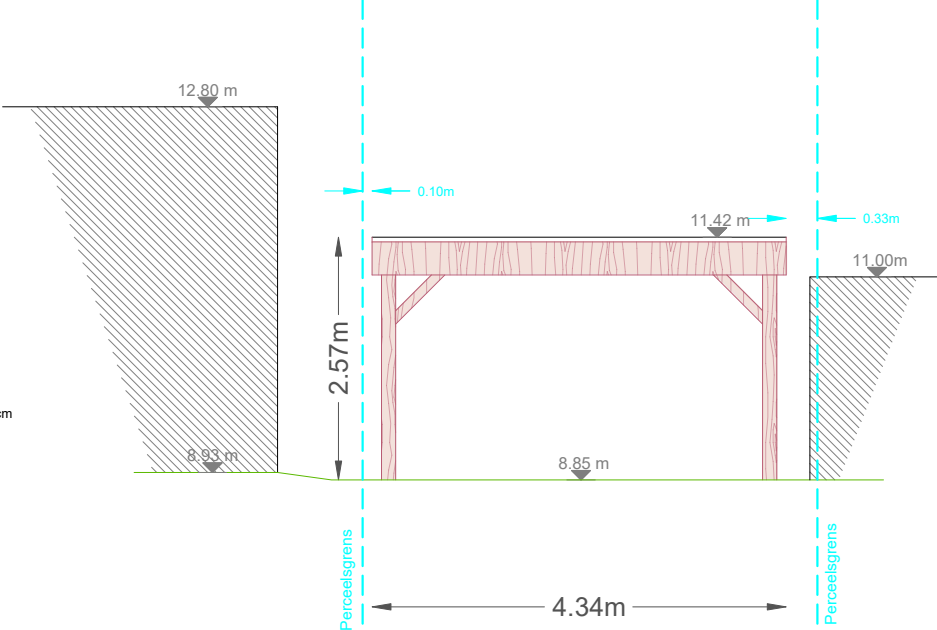
Carpot in hout met aluminium dakrand
