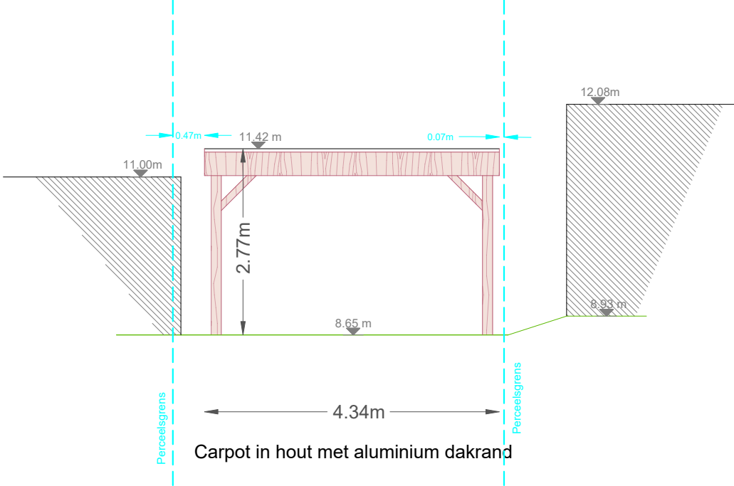
Carpot in hout met aluminium dakrand
