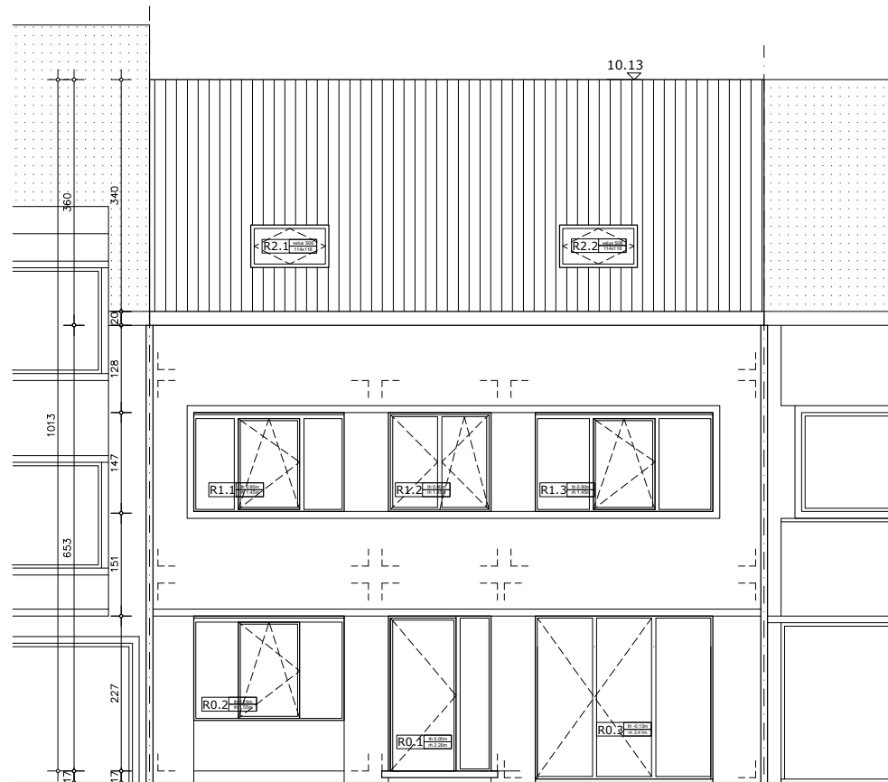
BESTAANDE TOESTAND VOORGEVEL 1-100
