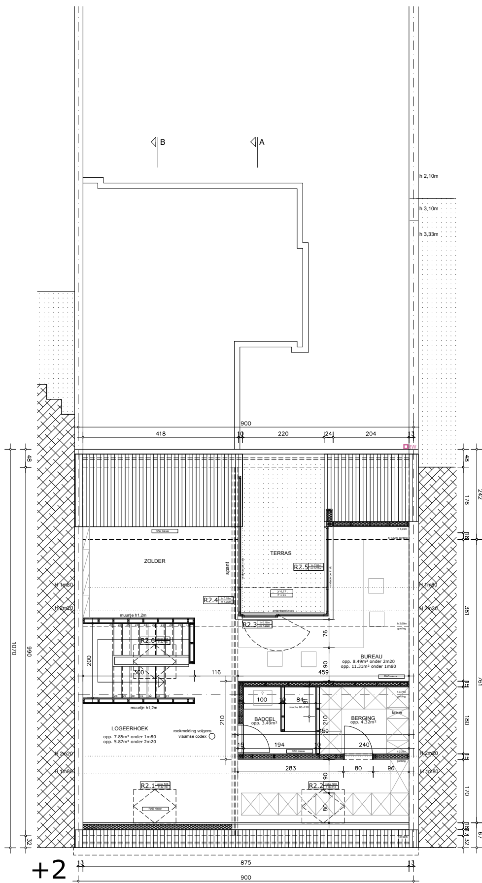
BESTAANDE TOESTAND TWEEDE VERDIEP 1-100
