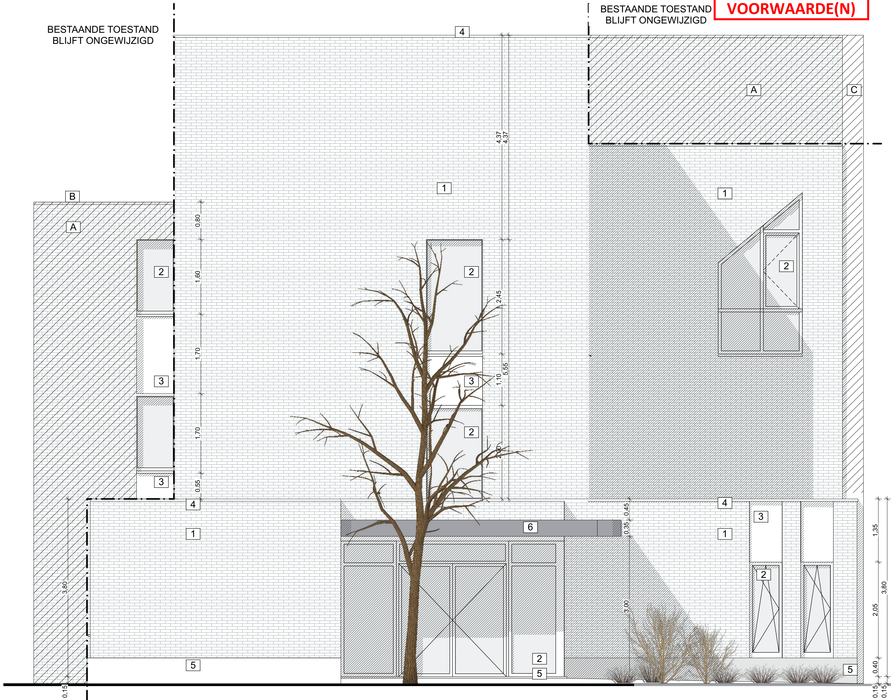
NIEUWE TOESTAND- GEVEL ZUID-OOST schaal 1/50, maataanduiding in meter.
