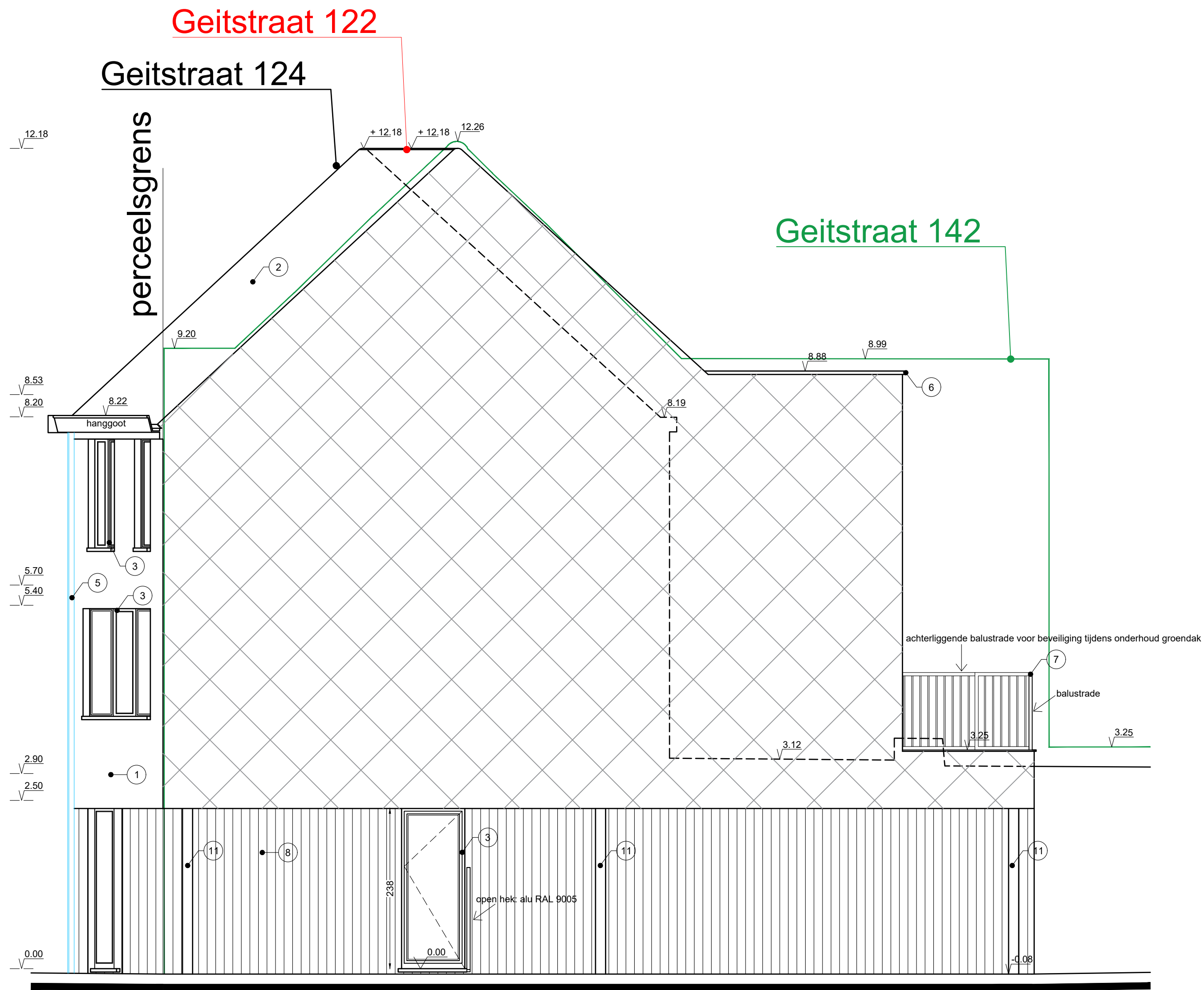
WONING - RECHTERZIJGEVEL NIEUWE TOESTAND
