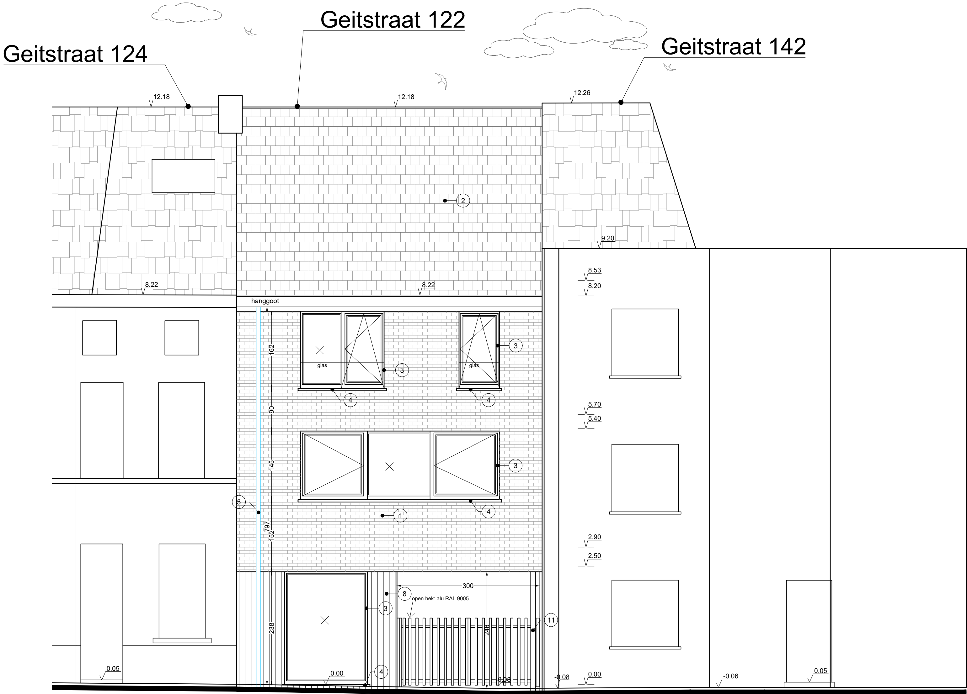
WONING - VOORGEVEL NIEUWE TOESTAND
