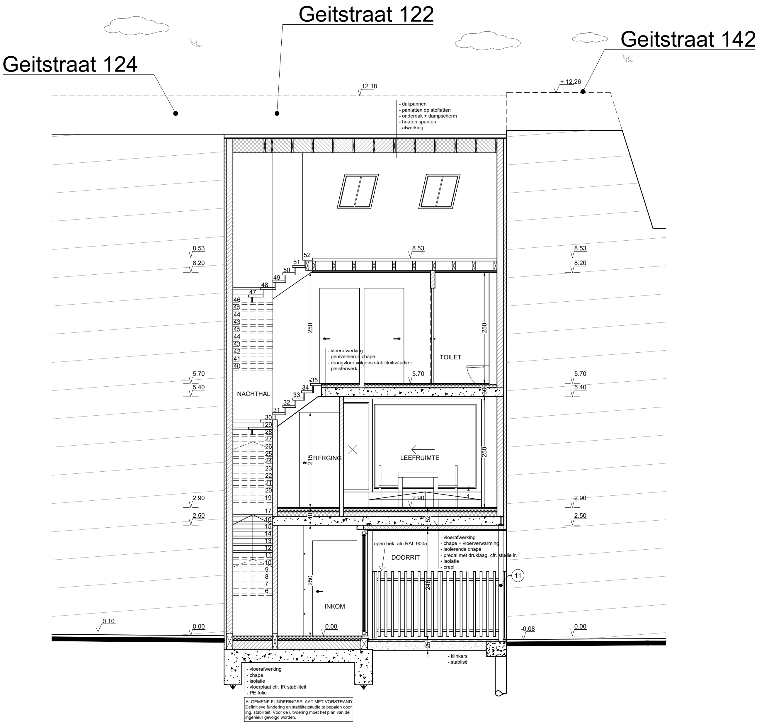
WONING - DOORSNEDE DD NIEUWE TOESTAND
