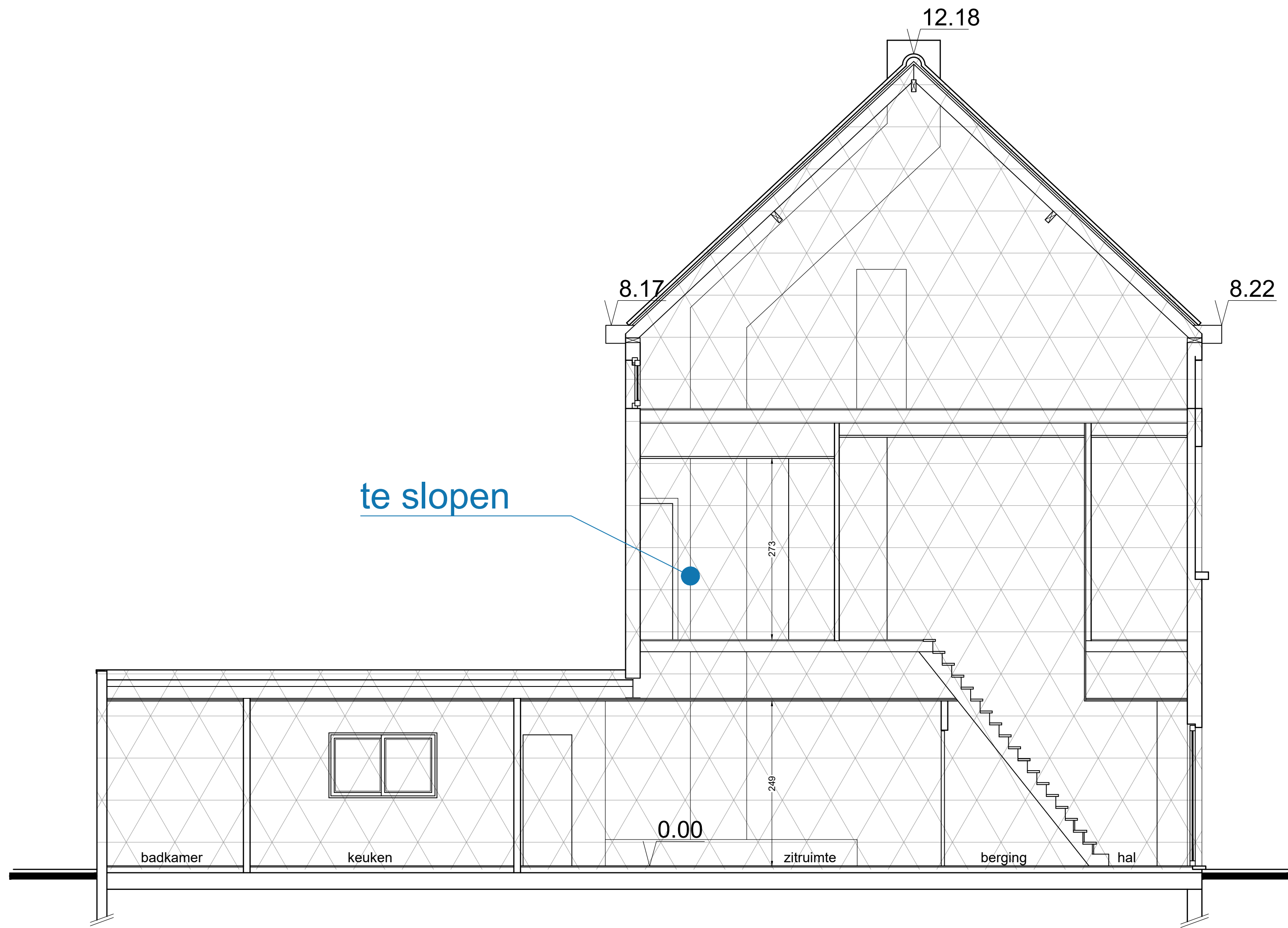
WONING - DOORSNEDE EE BESTAANDE TOESTAND - TE SLOPEN
