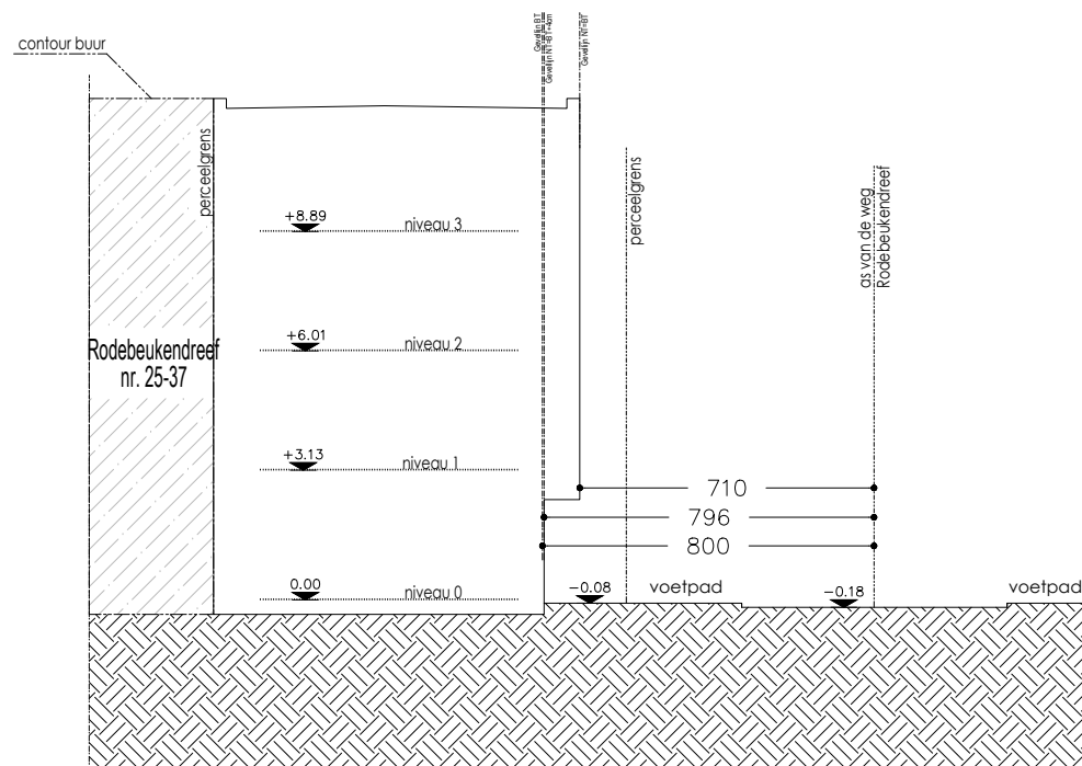
Terrein Profiel Nieuwe Toestand
