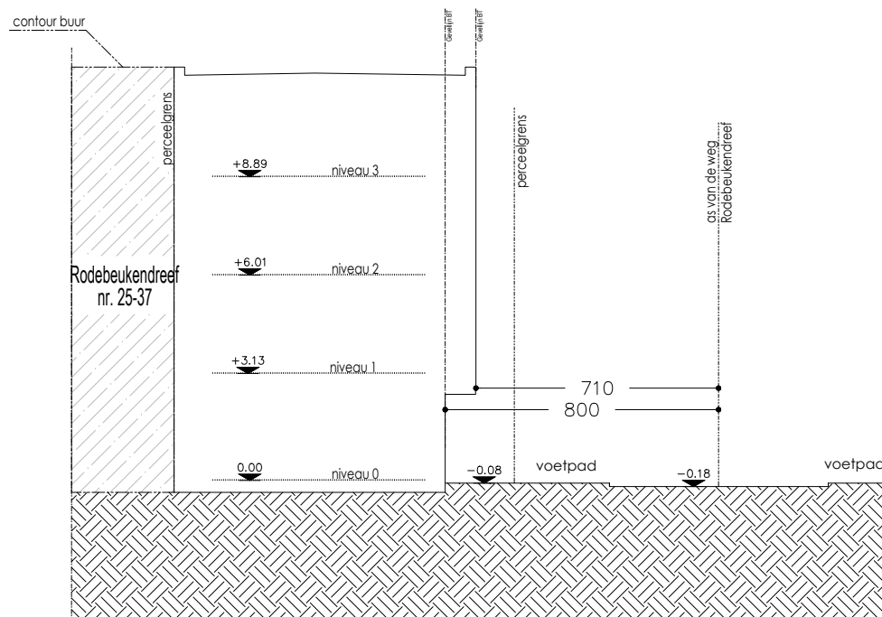
Terrein Profiel Bestaande Toestand
