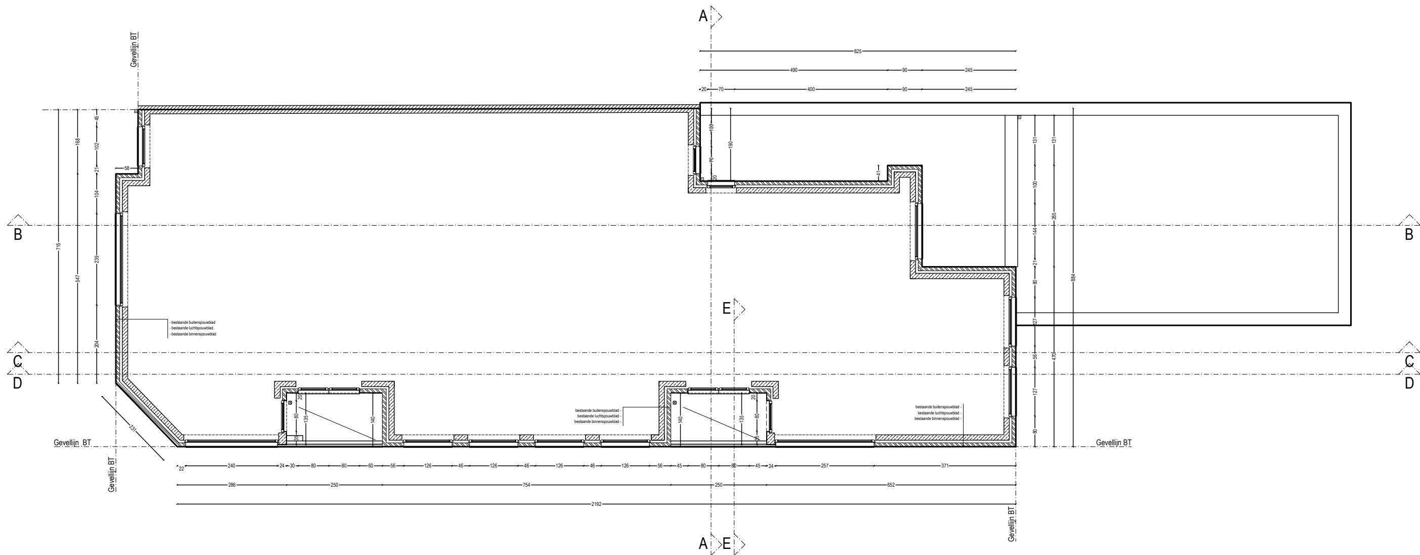
GRONDPLAN NIVEAU 1-3 BESTAANDE TOESTAND
