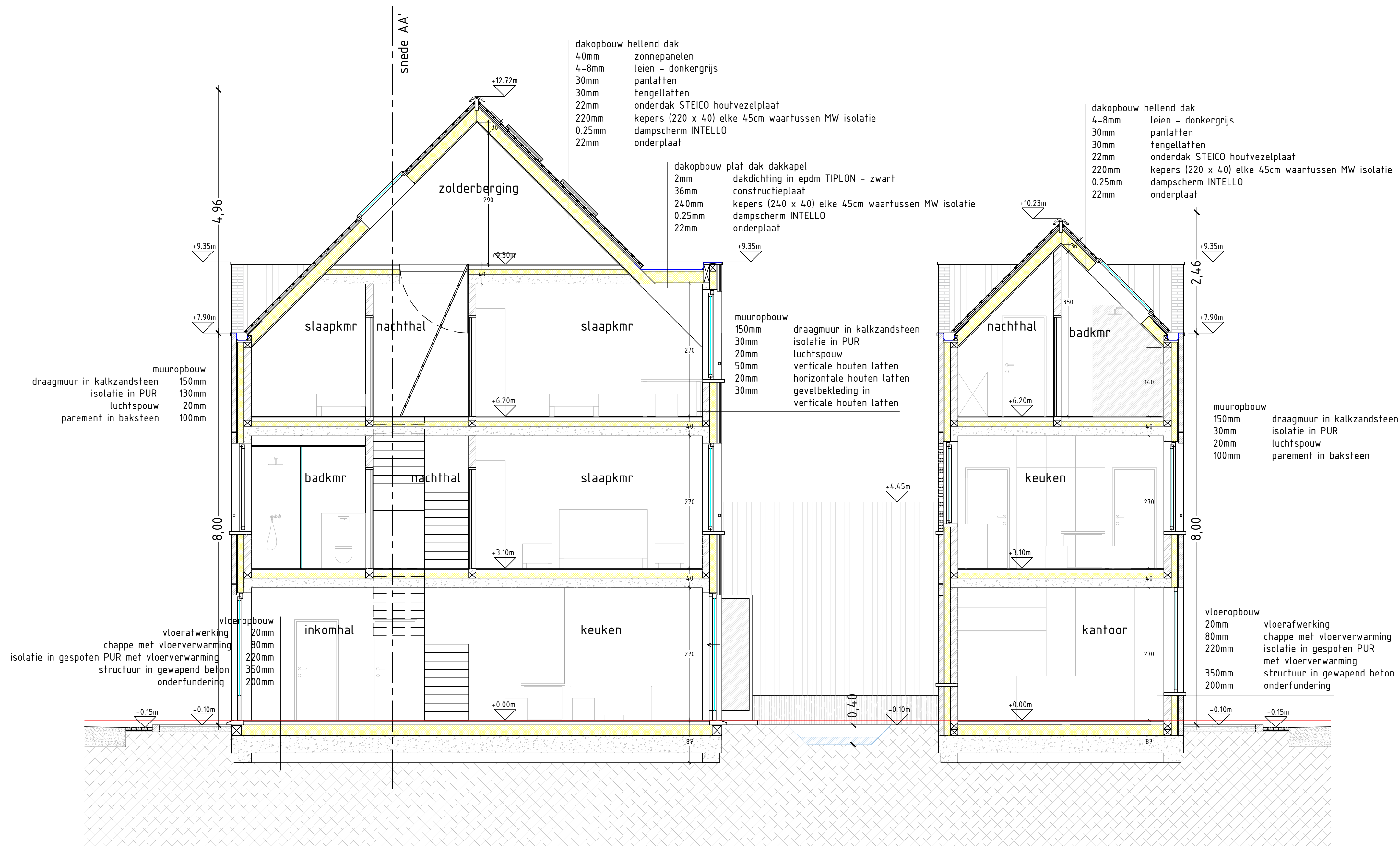
DOORSNEDE BB'
